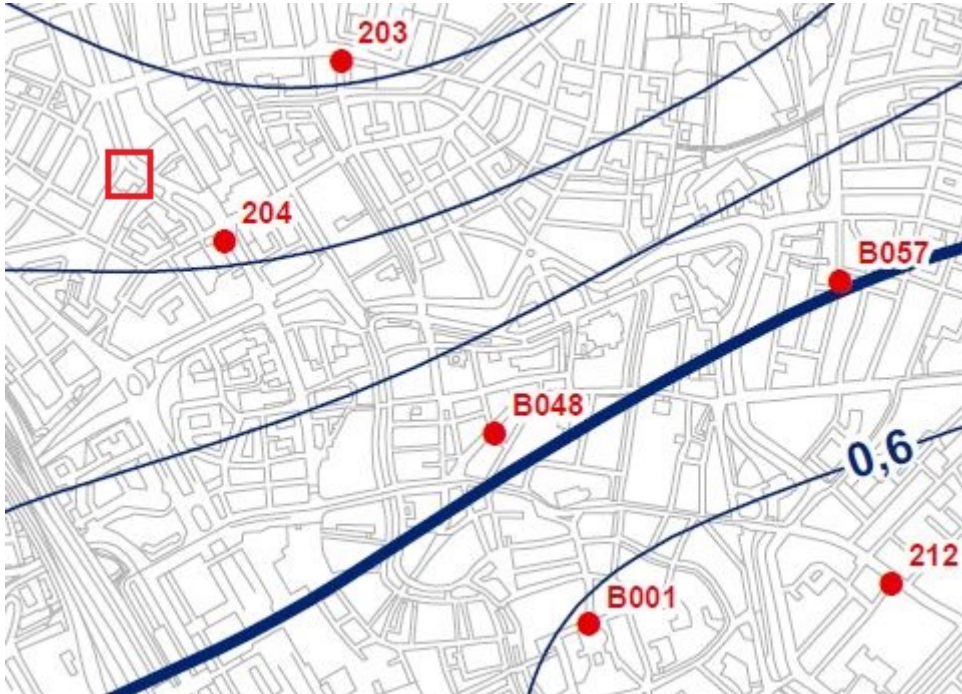
Figuur 5: Gemiddelde hoge grondwaterstand GHG (bron: Isohypsenaart gemeente Utrecht)
