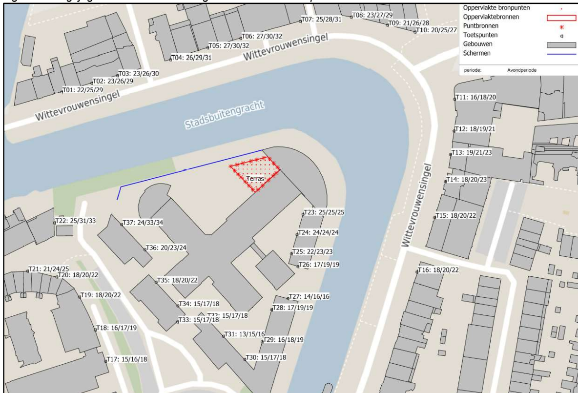
Figuur 3 Langtijdgemiddelde beoordelingsniveau in de avondperiode
