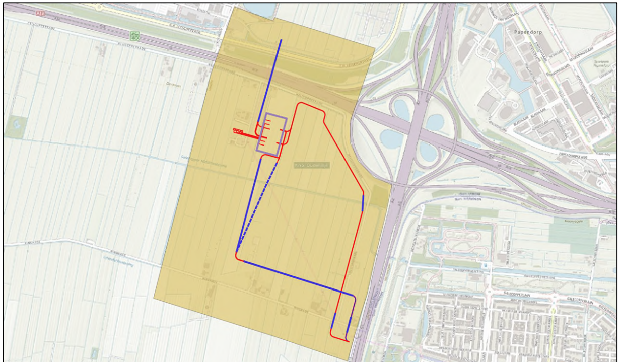
Figuur 1.2: Ligging onderzoeksgebied (gele arcering), de stationslocatie (paars omlijnd) en de tracé-varianten. De aanlegmethode in de tracés is weergegeven, met in rood veldstrekking en in blauw horizontaal gestuurde boringen (HDD's). De blauw gestippelde HDD is een subvariant en één van de tracévarianten. Bron ondergrond: TopoPlus.
