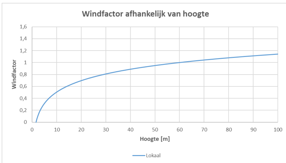
Figuur 6: Toegepast windprofiel.
