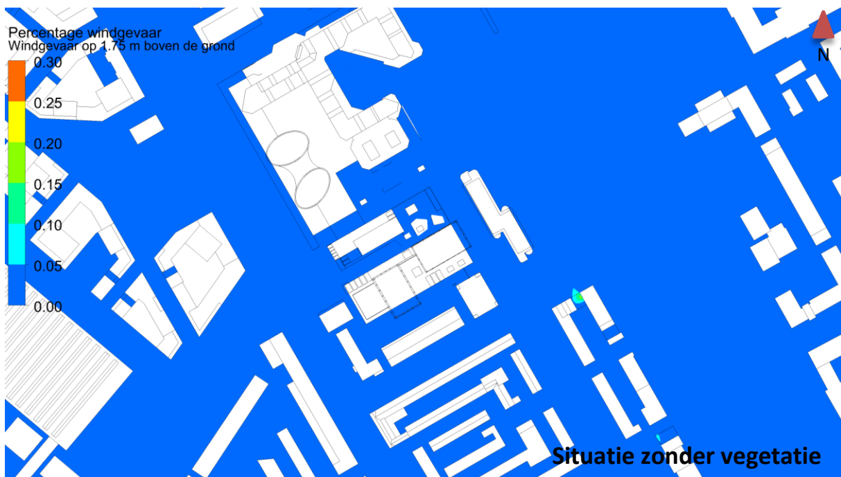
Figuur 12: Percentage windgevaar per jaar op 1,75 m boven de grondvlakken voor de situatie zonder vegetatie.
