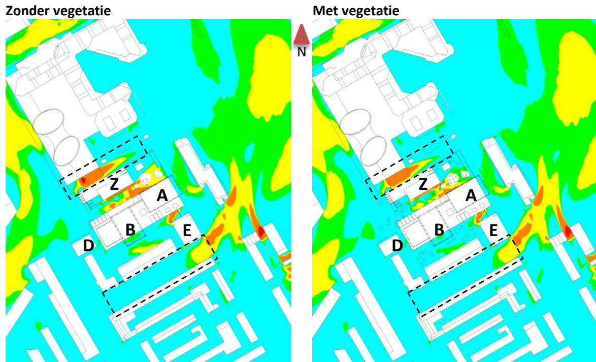
Figuur 11: Kwaliteitsklasse op 1,75 meter boven straatniveau volgens de NEN 8100.
