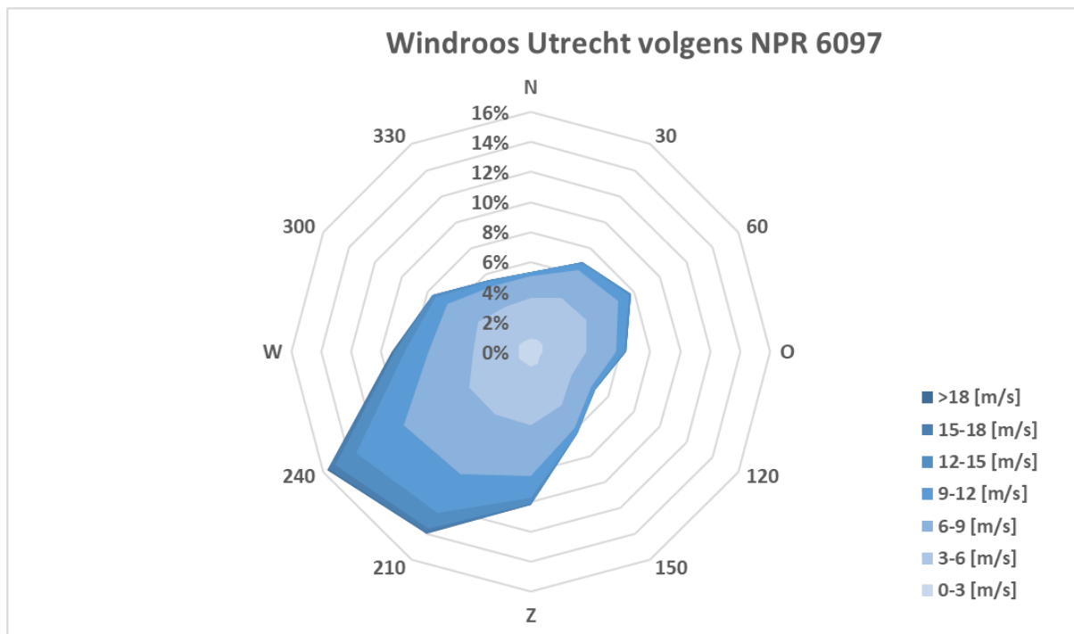
Figuur 4: Windroos Utrecht, volgens NPR 6097.
