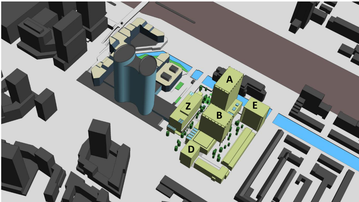
Figuur 2: 3D model van het bestuurscentrum van de Rabobank met vegetatie. De gebouwen gekleurd in het olijfgroen behoren tot de herontwikkeling Matserterein. De donkergroene delen tonen de locaties van de vegetatie.
