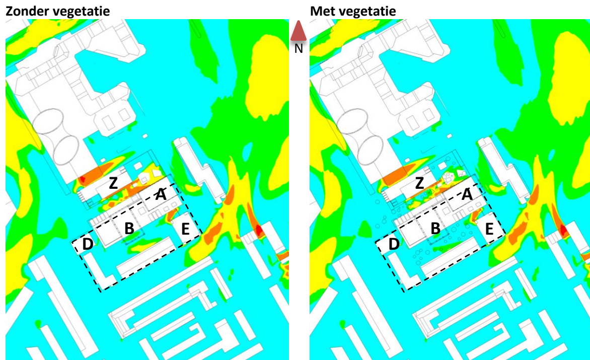
Figuur 10: Kwaliteitsklasse op 1,75 meter boven straatniveau volgens de NEN 8100.
