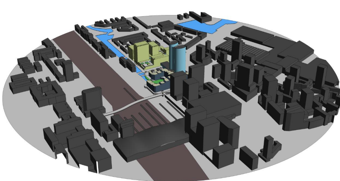
Figuur 3: Overzicht van het 3D CFD model. De gebouwen gekleurd in het olijfgroen behoren tot de herontwikkeling Matsertterrein.
