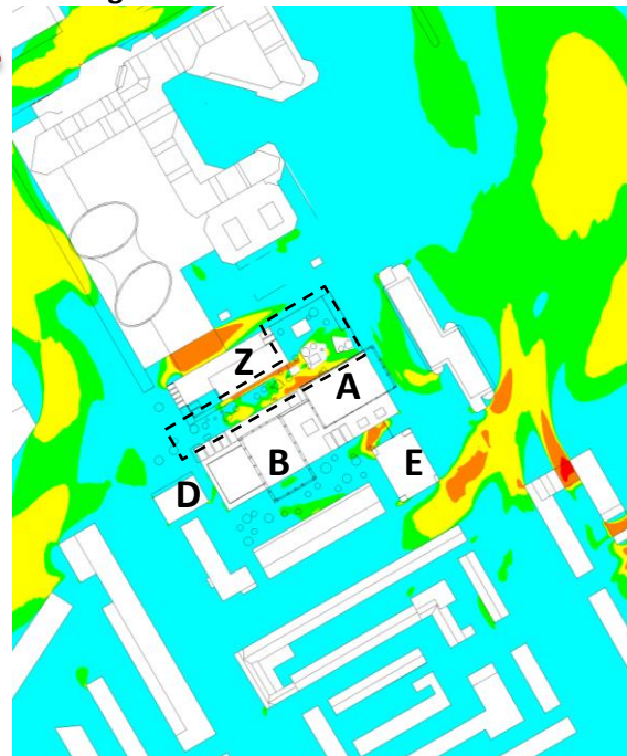
Figuur 9: Kwaliteitsklasse op 1,75 meter boven straatniveau volgens de NEN 8100.
