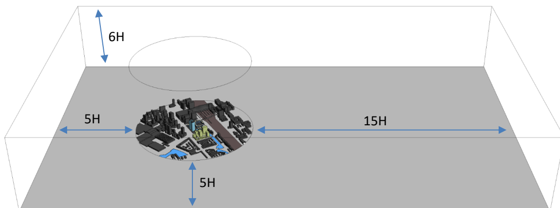
Figuur 5: Winddomein om het gemodelleerde gebied heen, ten behoeve van het windprofiel (digitale windtunnel).
