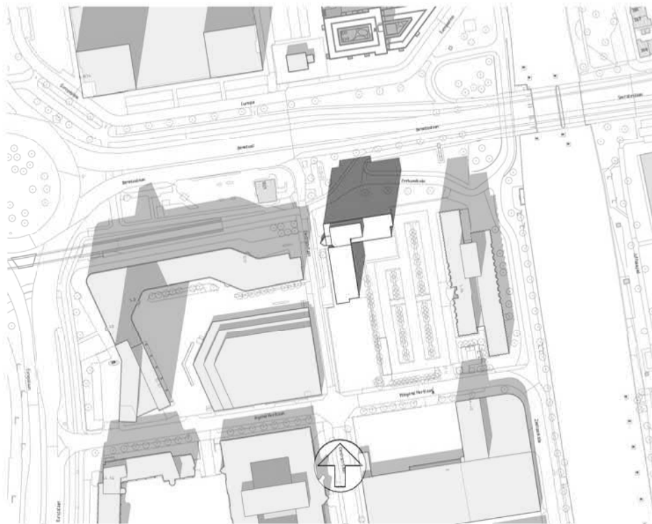
21 september 14.00uur
