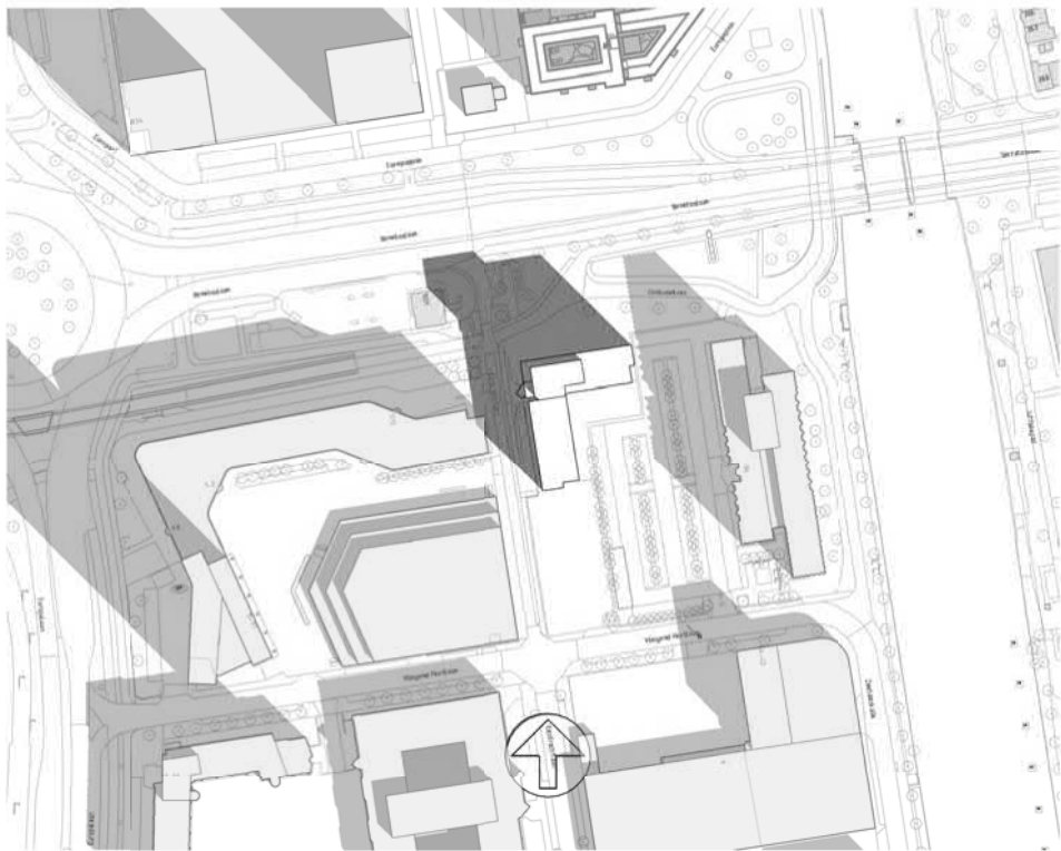
21 september 11.00uur
