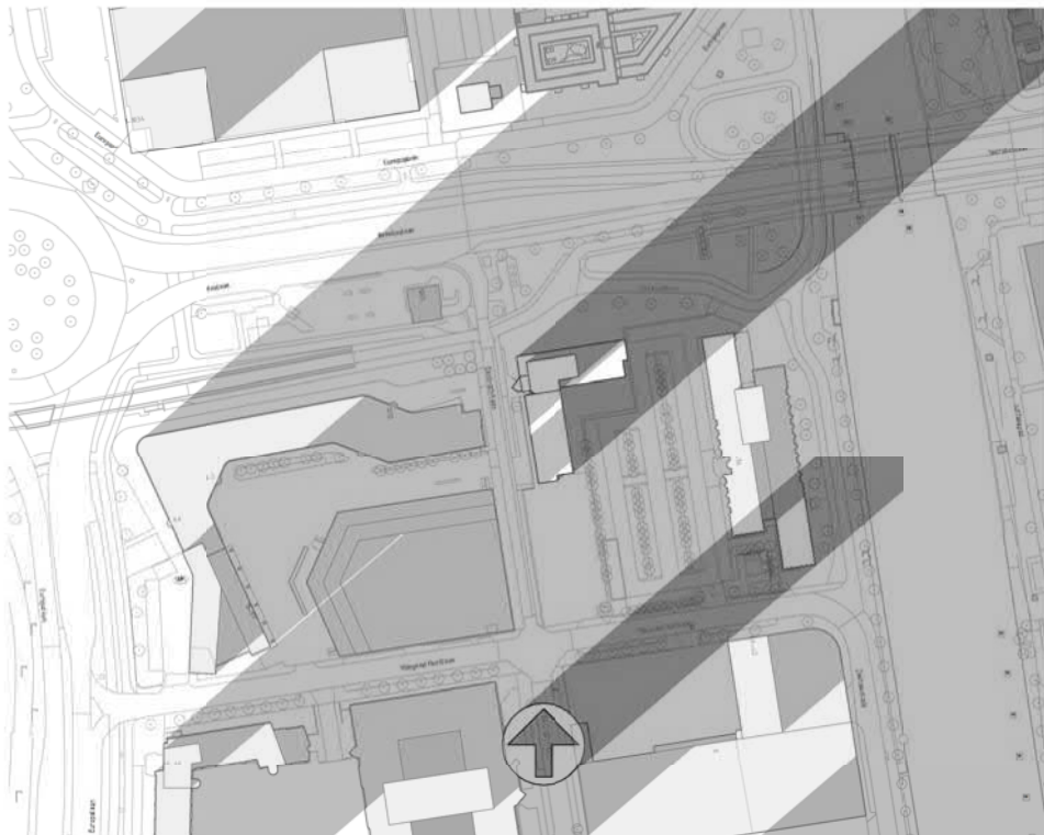
21 december 18.00uur
