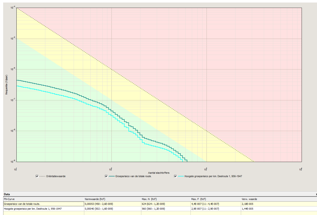
Grafiek 3.1: fN-curve berekend groepsrisico huidige situatie
