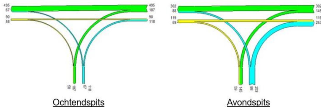
Afbeelding 20: kruispuntstromen
