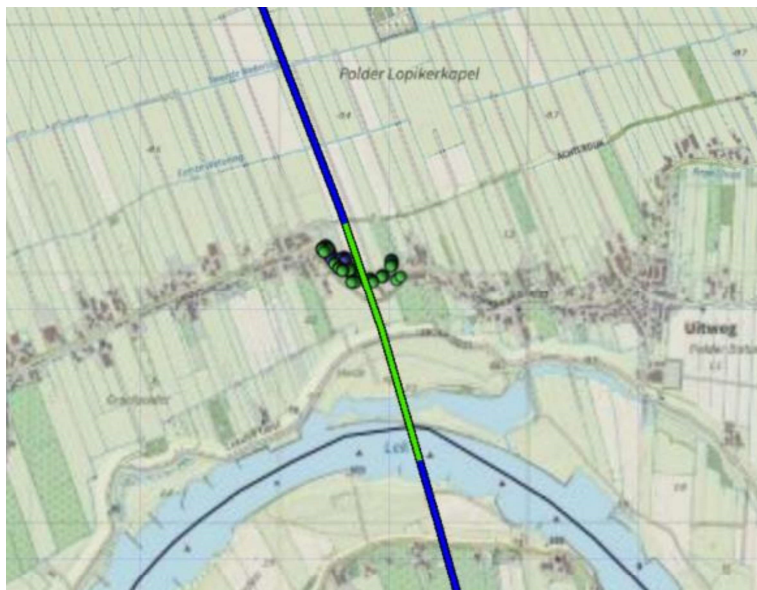
Figuur 28: Kilometer met hoogste groepsrisico aardgasleiding A-555-08 gemeente Lopik
