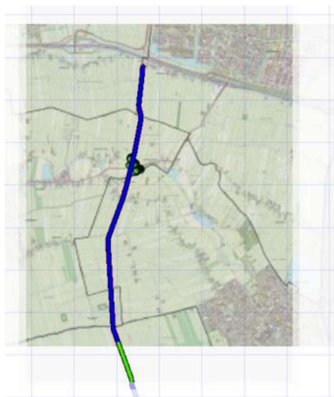
Figuur 20: Kilometer met hoogste groepsrisico aardgasleiding A-555-08-deel-1 gemeente Montfoort
