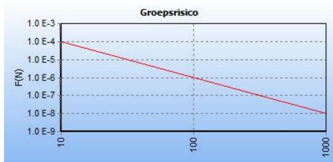
Figuur 18: Groepsrisico aardgasleiding A-555-08 gemeente Utrecht
