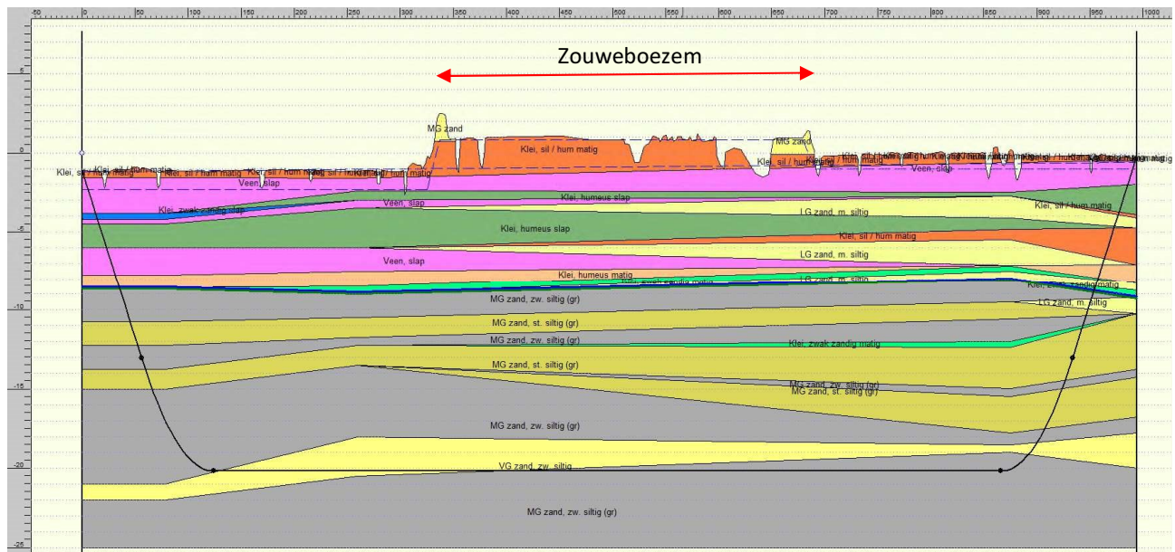
Figuur 2.3: langprofiel HDD onder Natura 2000-gebied Zouweboezem
