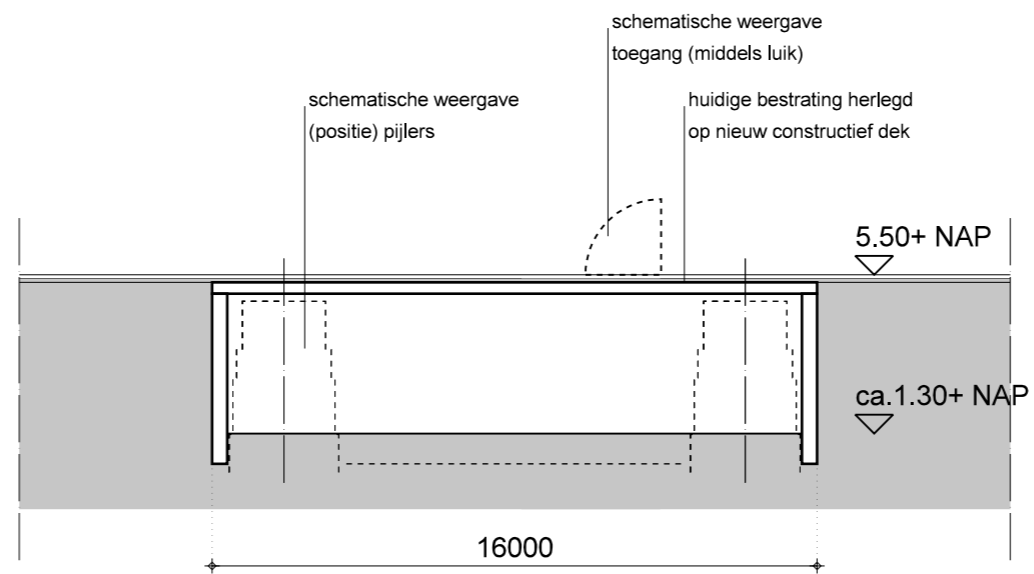
LANGSDOORSNEDE
