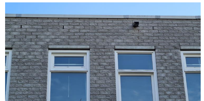
Figuur 9: Detail westzijde gebouw met openstootvoegen en kierende dakrand
