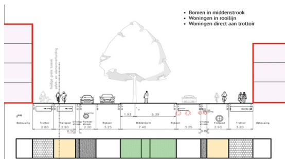
Illustratie: vastgesteld Voorlopig Ontwerp 17 november 2020: Tekening versmallen Croeselaan. Het smalle profiel van de Croeselaan wordt op een logische manier doorgetrokken naar de kruising met de Van Zijstweg, waar het profiel zich verbreedt; wegen, fietspaden en trottoirs worden op een logische manier op elkaar aangesloten.
