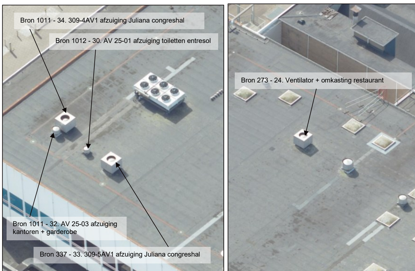
Figuur 9 Overzicht ligging geluidsbronnen Jaarbeurs ter hoogte van gebouwen 1C en 1D
