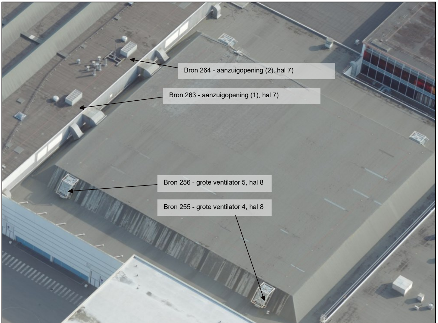
Figuur 10 Overzicht ligging maatgevende geluidsbronnen Jaarbeursgebouw 2A t/m 2D
