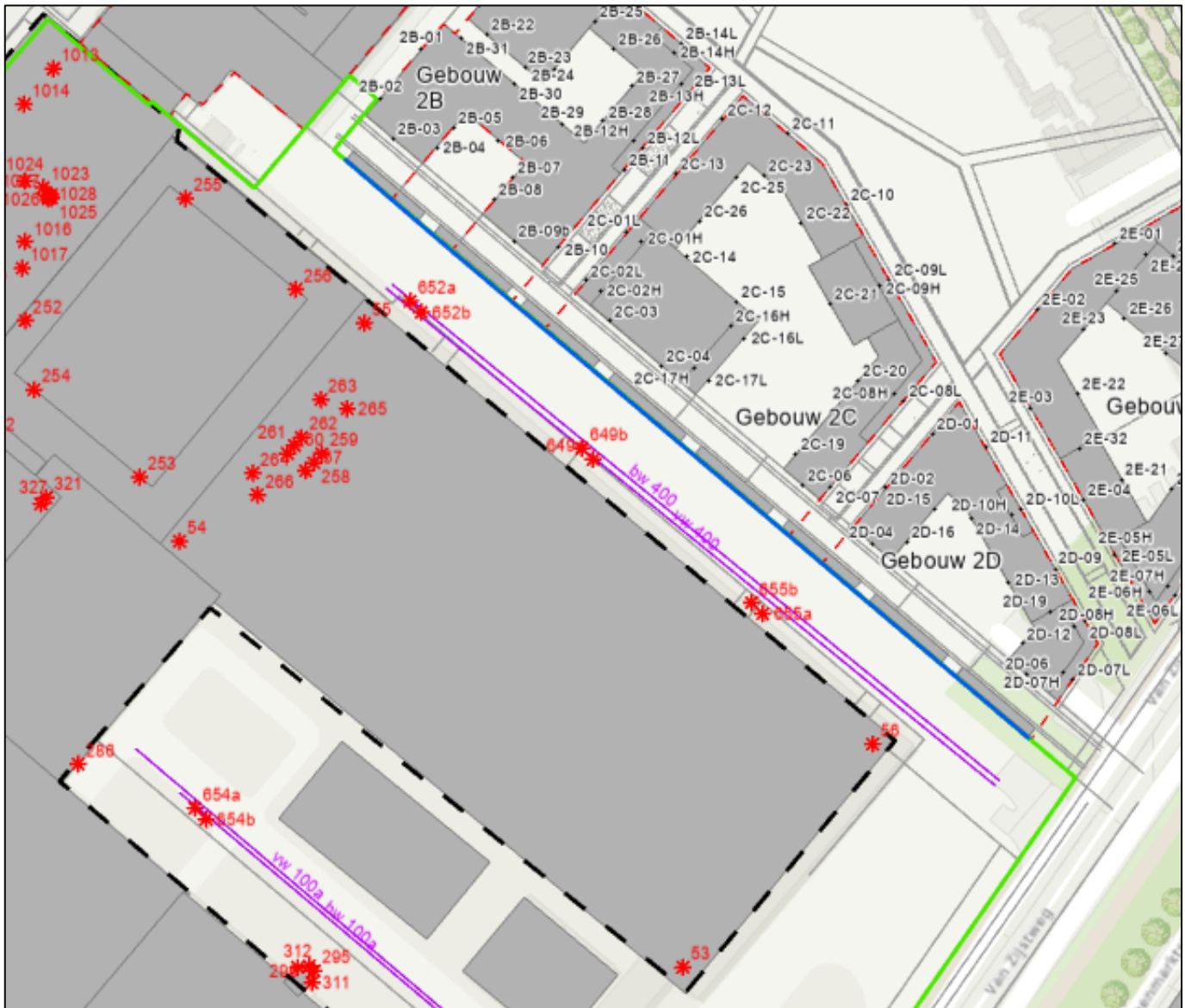
Figuur 8 Overzicht ligging 3 lagen containers met openingen als maatregel (uitgangspunt SP, in model als 7,5 m hoog scherm) en ligging bronnen en rekenpunten
