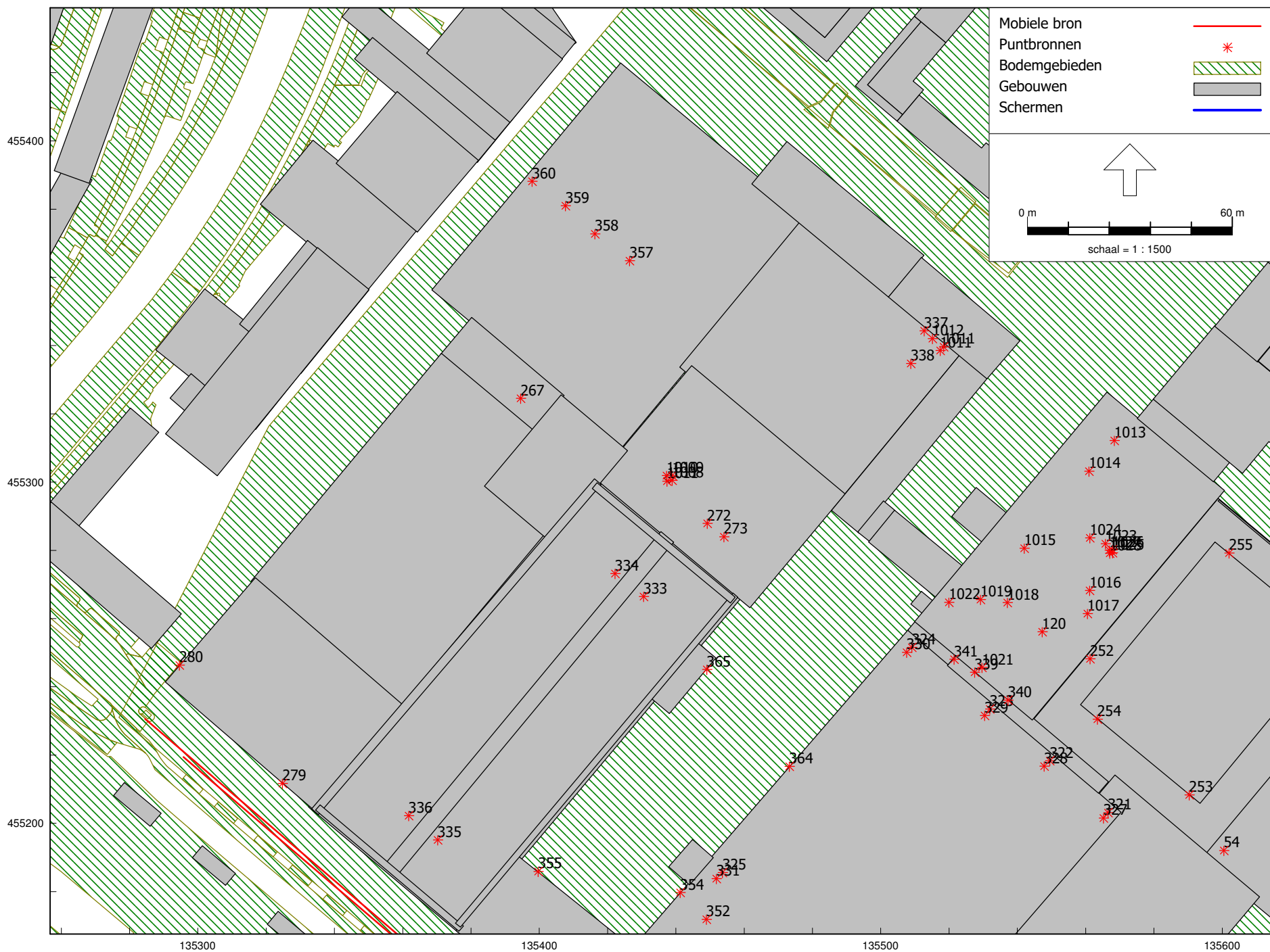
Overzicht ligging puntbronnen en mobiele bronnen Jaarbeurs - opbouw beurs
