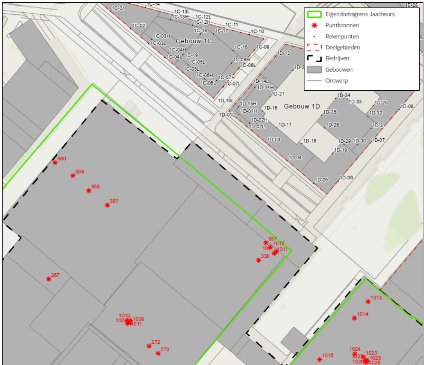
Figuur 7 Overzicht ligging gebouwen 1C en 1D, rekenpunten gebouwen en geluidbronnen
