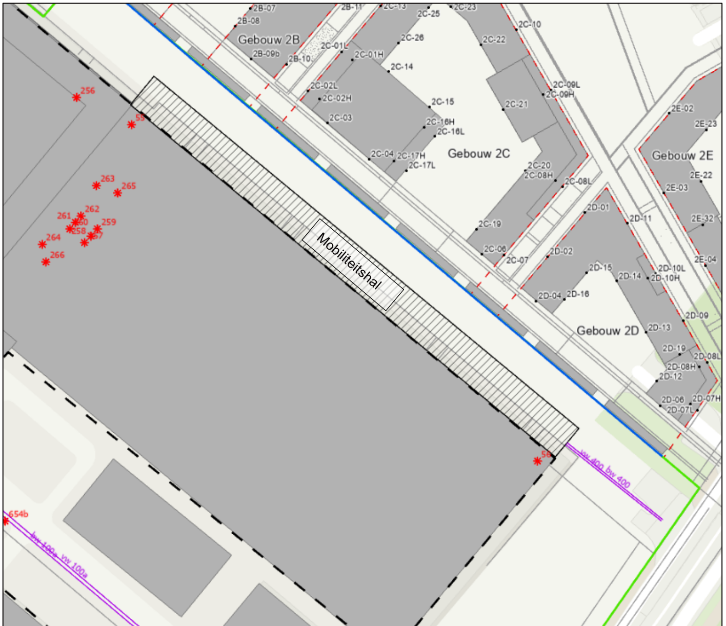
Figuur 12 Voorbeeld locatie aanbouw hal t.b.v. laden/lossen transport en locatie containers/geluidsscherm 6,5m+
