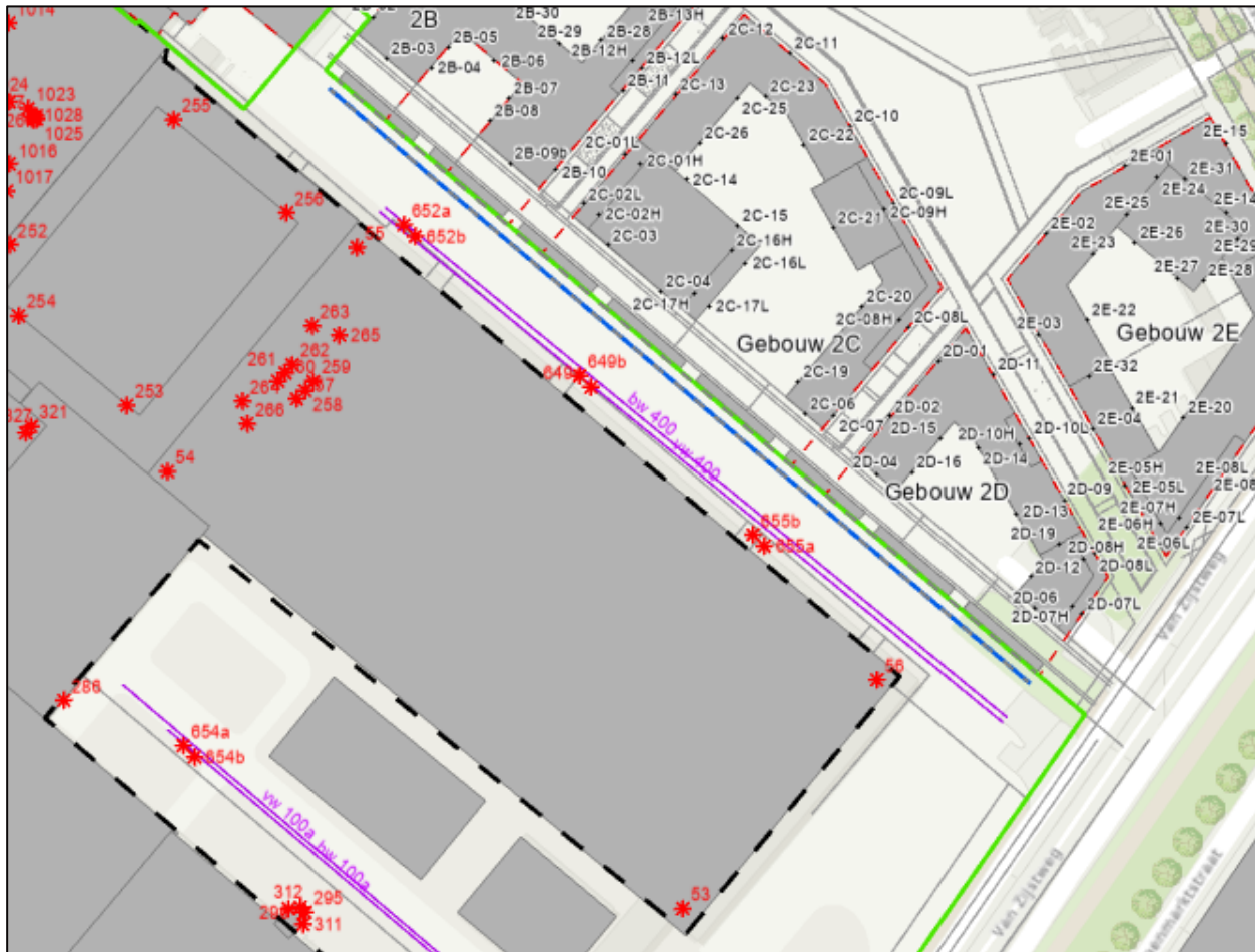
Figuur 11 Overzicht ligging 3 lagen containers met openingen als maatregel (uitgangspunt SP) in model en absorberend scherm van in totaal 12 m hoog op grens terrein, waarvan 7,5 m hoog rechtstand en 4,5 m hoog onder een hoek, waardoor de top 3m teruggebogen wordt richting Jaarbeurs
