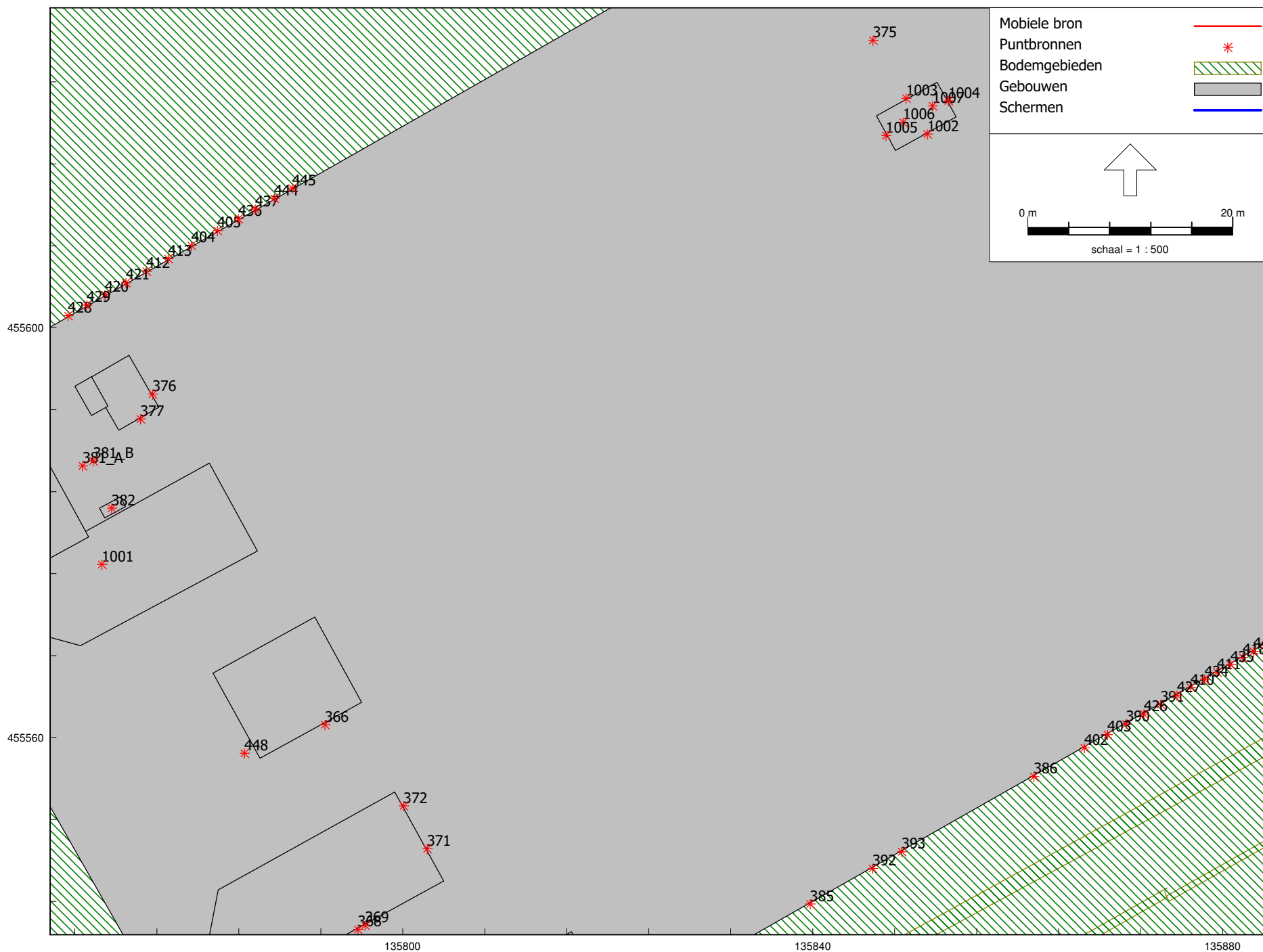
Overzicht ligging puntbronnen en mobiele bronnen
