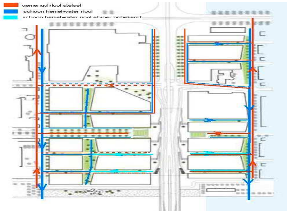
afbeelding 4.1 principe afwateringssysteem
