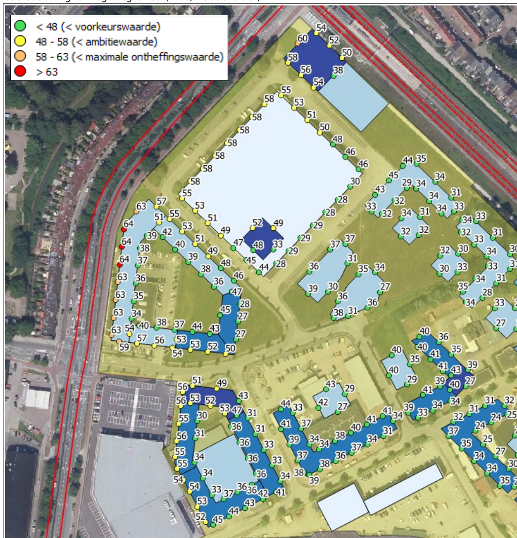
f4.2 Geluidbelasting vanwege wegverkeer (in dB, inclusief aftrek).
