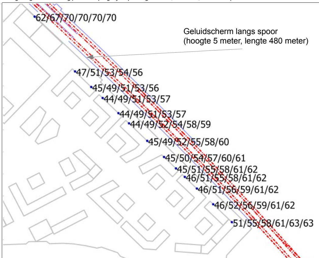
f5.4 Weergave geluidbelasting per verdieping bij toepassing scherm (h=5meter) en raildempers.
