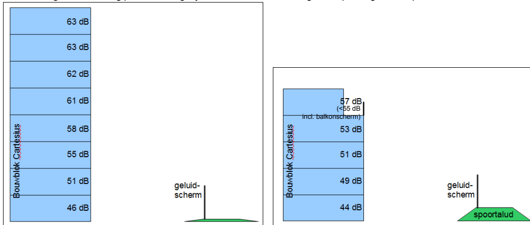
f5.3 Doorsnede geluidbelasting per bouwlaag bij scherm van 5 meter hoog en toepassing raildempers.
