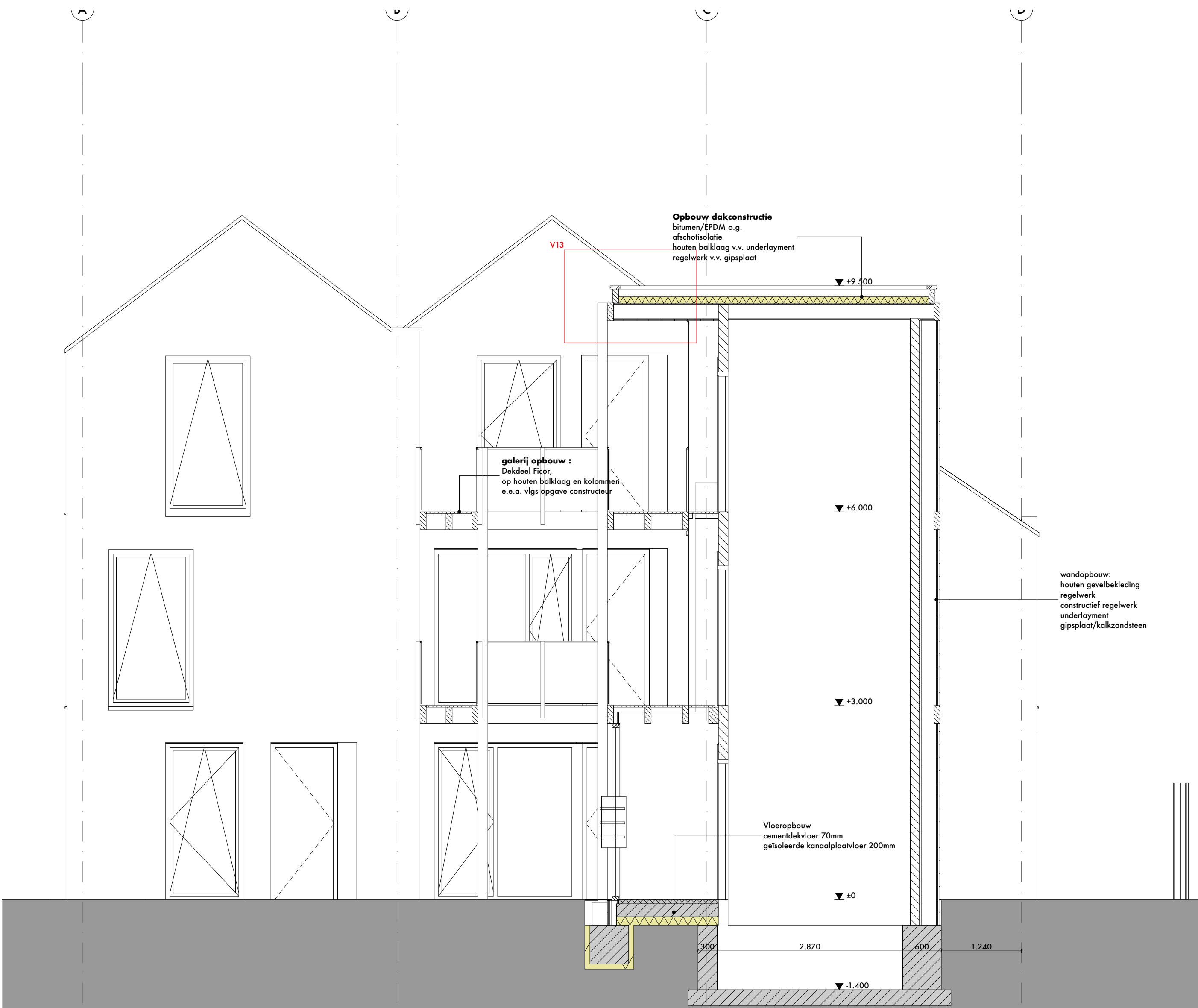
Doorsnede E-E 1:50
