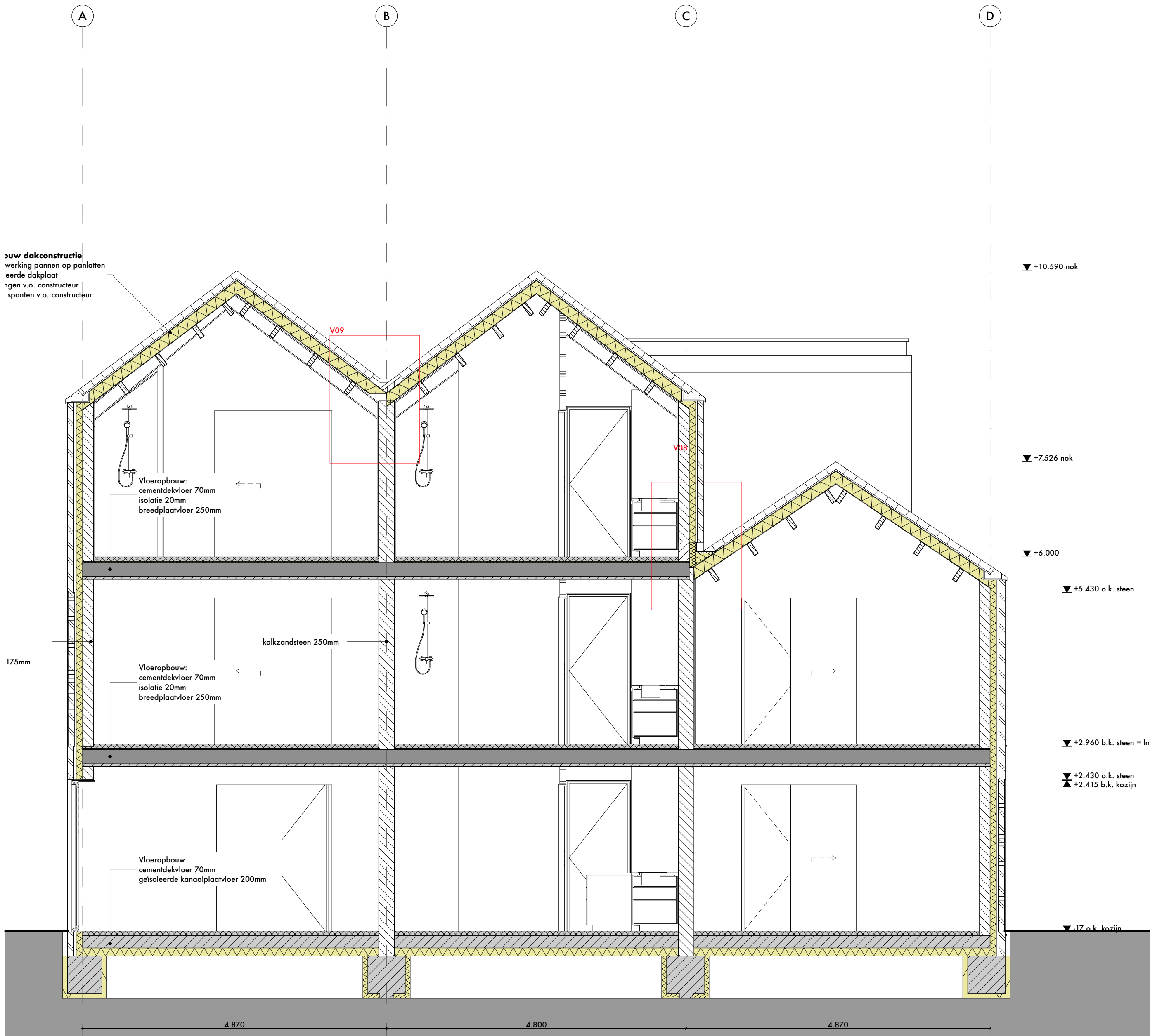
Doorsnede C-C 1:50
