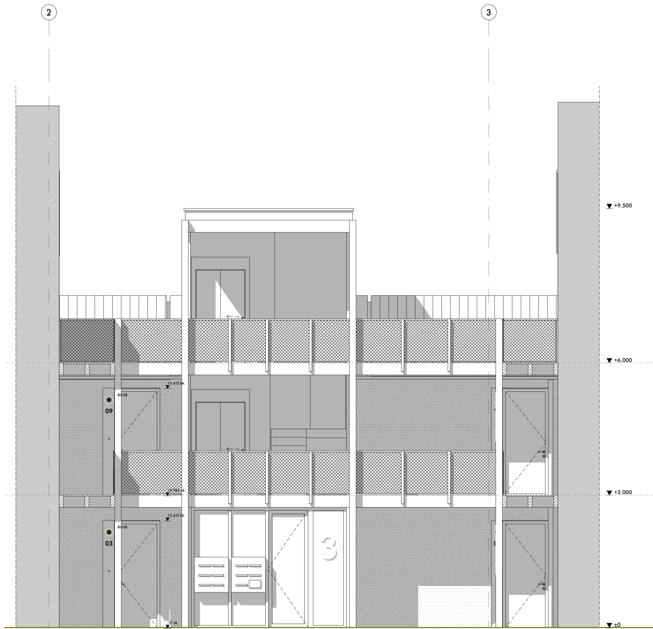
Linkerzijgevel as C 1:50
