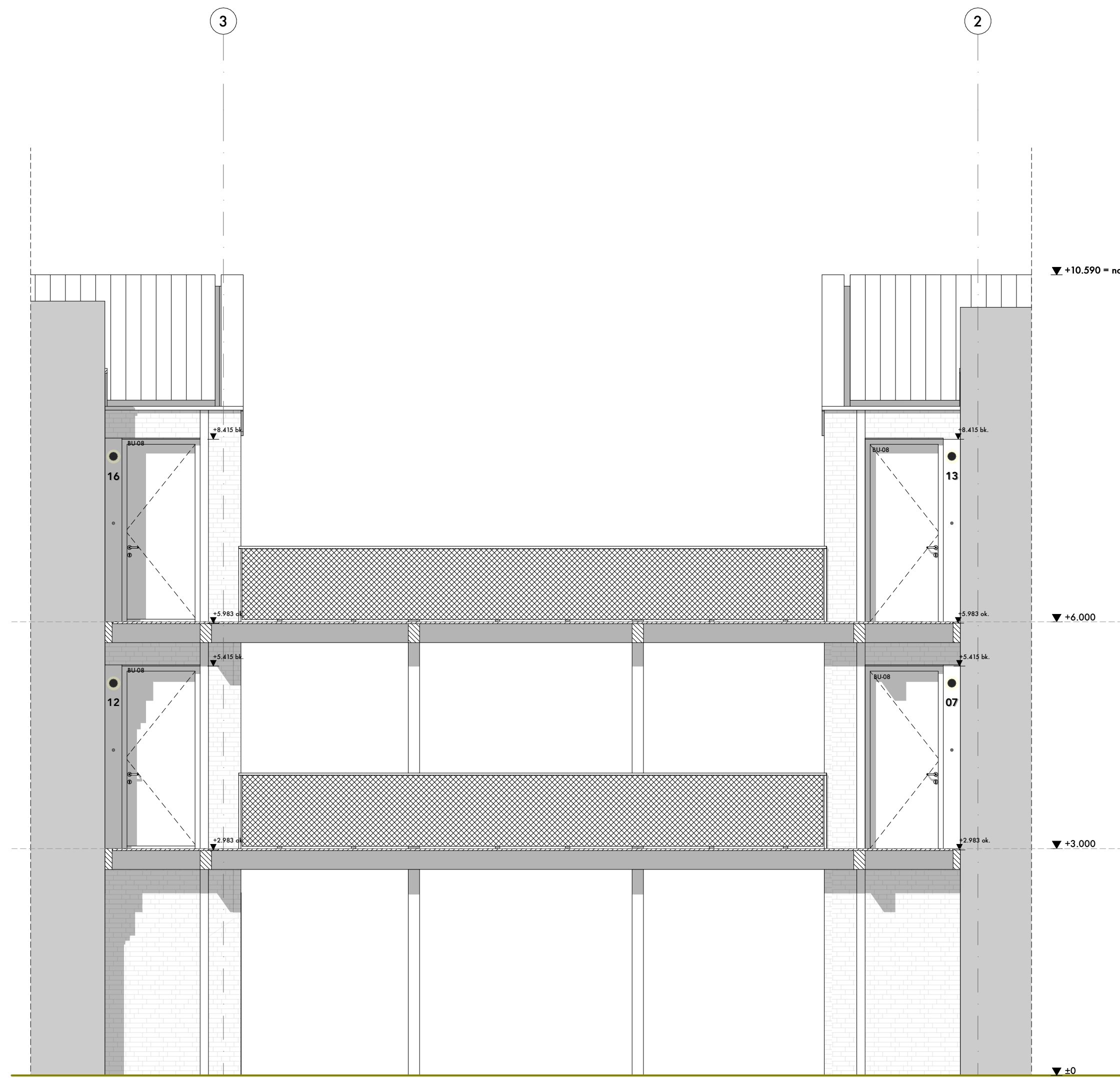
Linkerzijgevel as B 1:50
