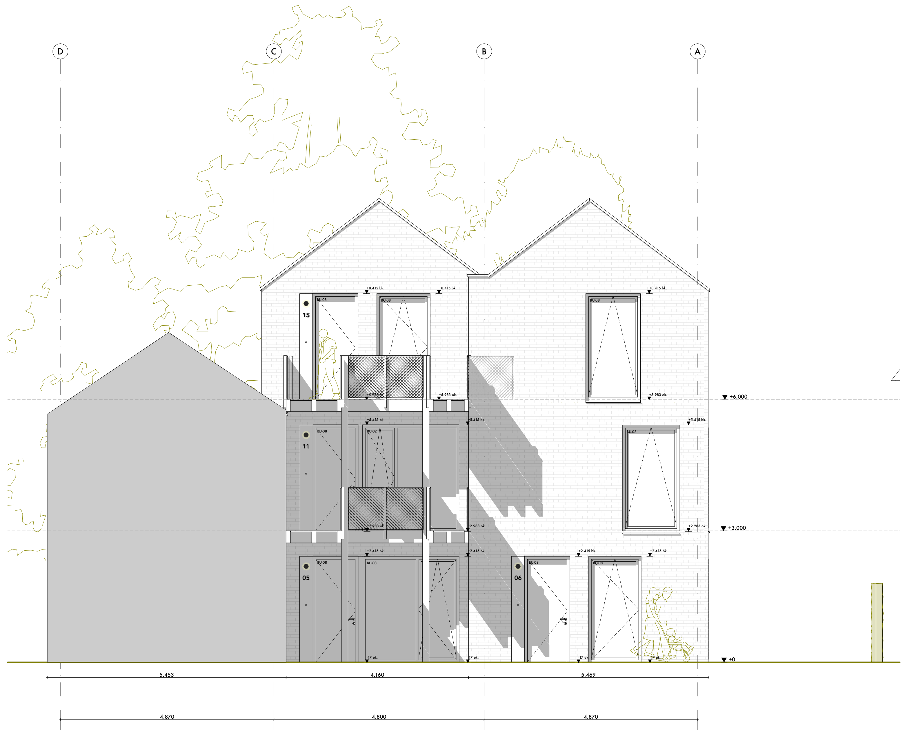
Binnengevel as3 1:50
