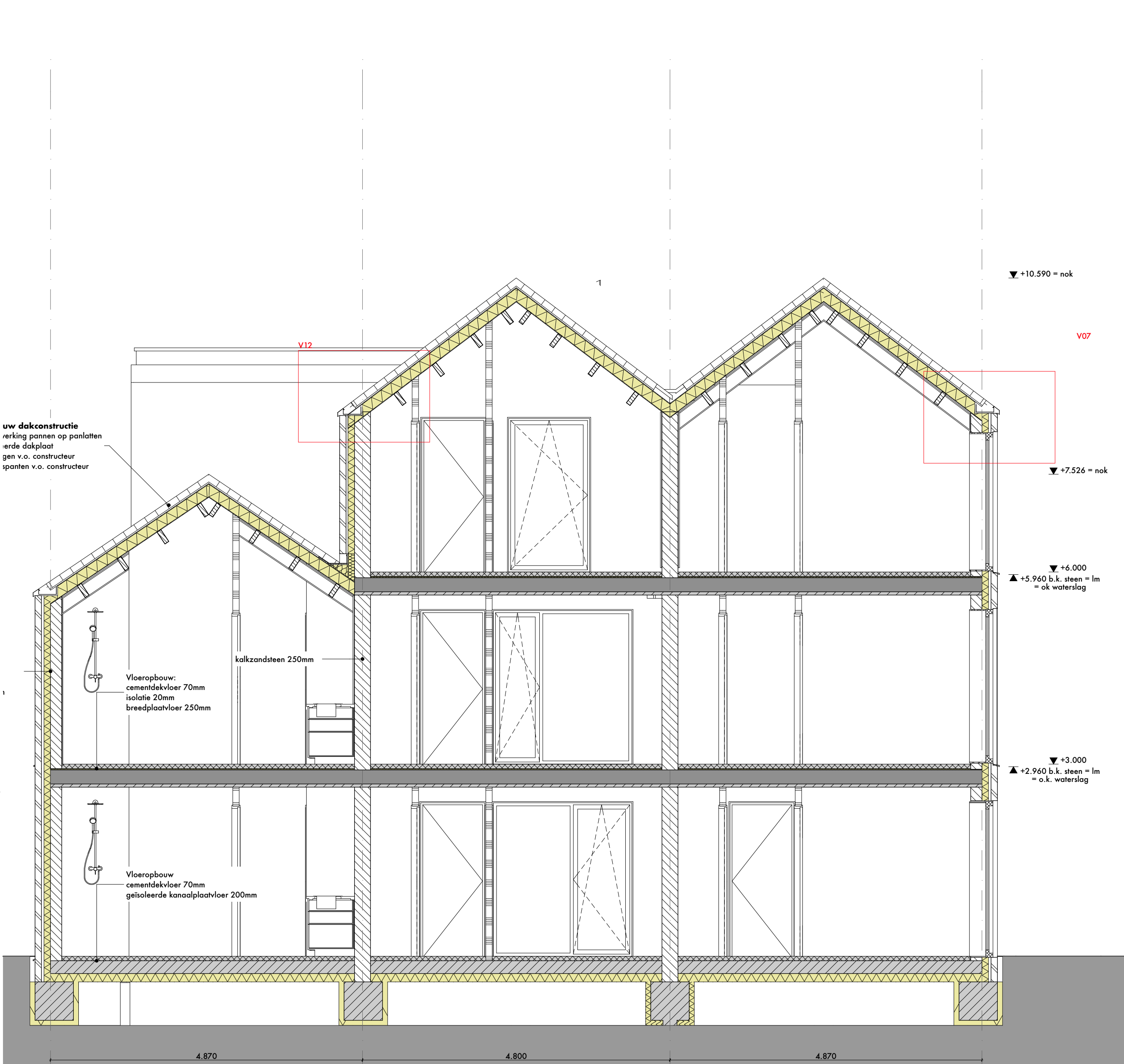
Doorsnede B-B 1:50
