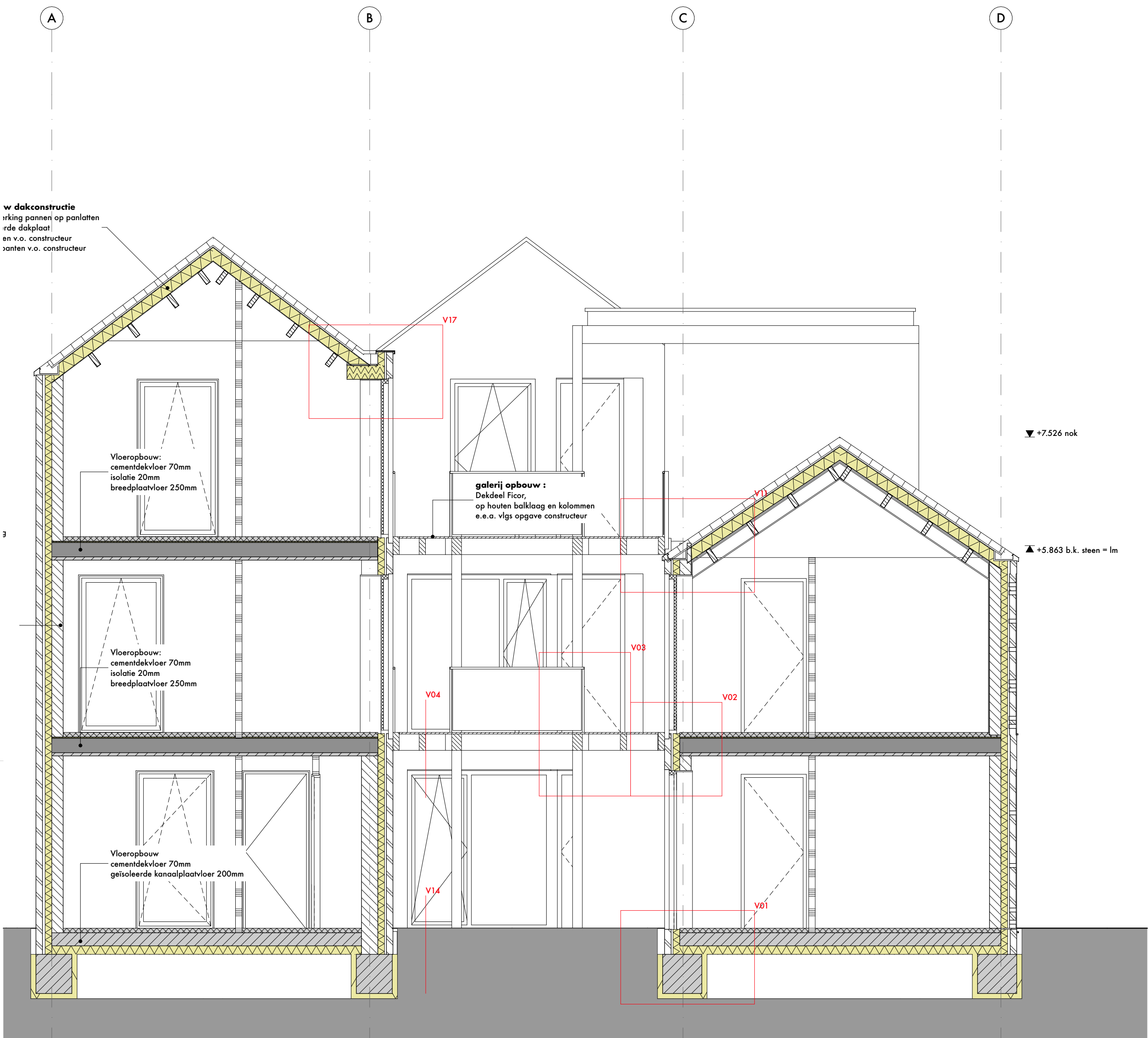
Doorsnede D-D 1:50
