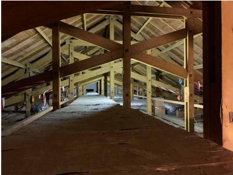
Foto – bestaande spantconstructie
