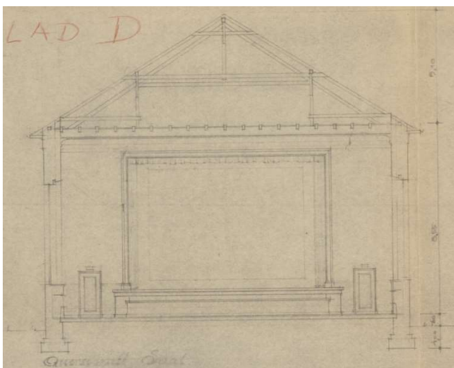
Tekening – fragment bouwtekening met doorsnede Großer Saal
