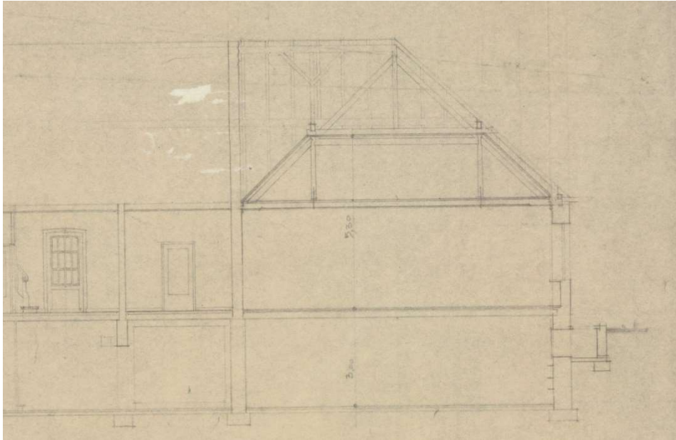
Tekening – fragment bouwtekening met doorsnede kop zijvleugel
