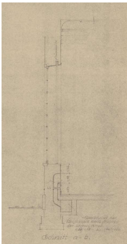
Doorsnede – detail van oorspronkelijke verwarming grote zaal
