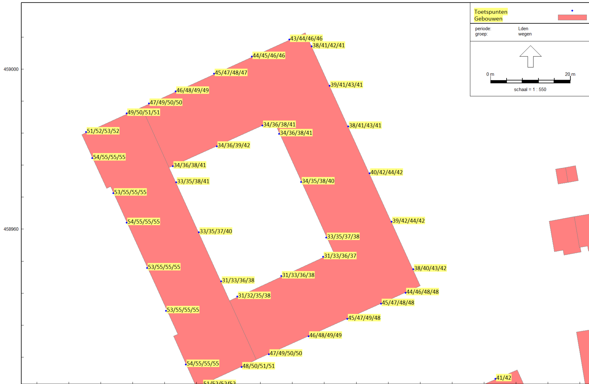
Figuur 6 Gebouw A: Gecumuleerde geluidsbelastingen vanwege wegverkeer op de omliggende wegen exclusief 2 en 5 dB correctie conform artikel 110g Wgh Beoordelingshoogte 1,5 / 4,5 / 7,5 en 10,5 meter
