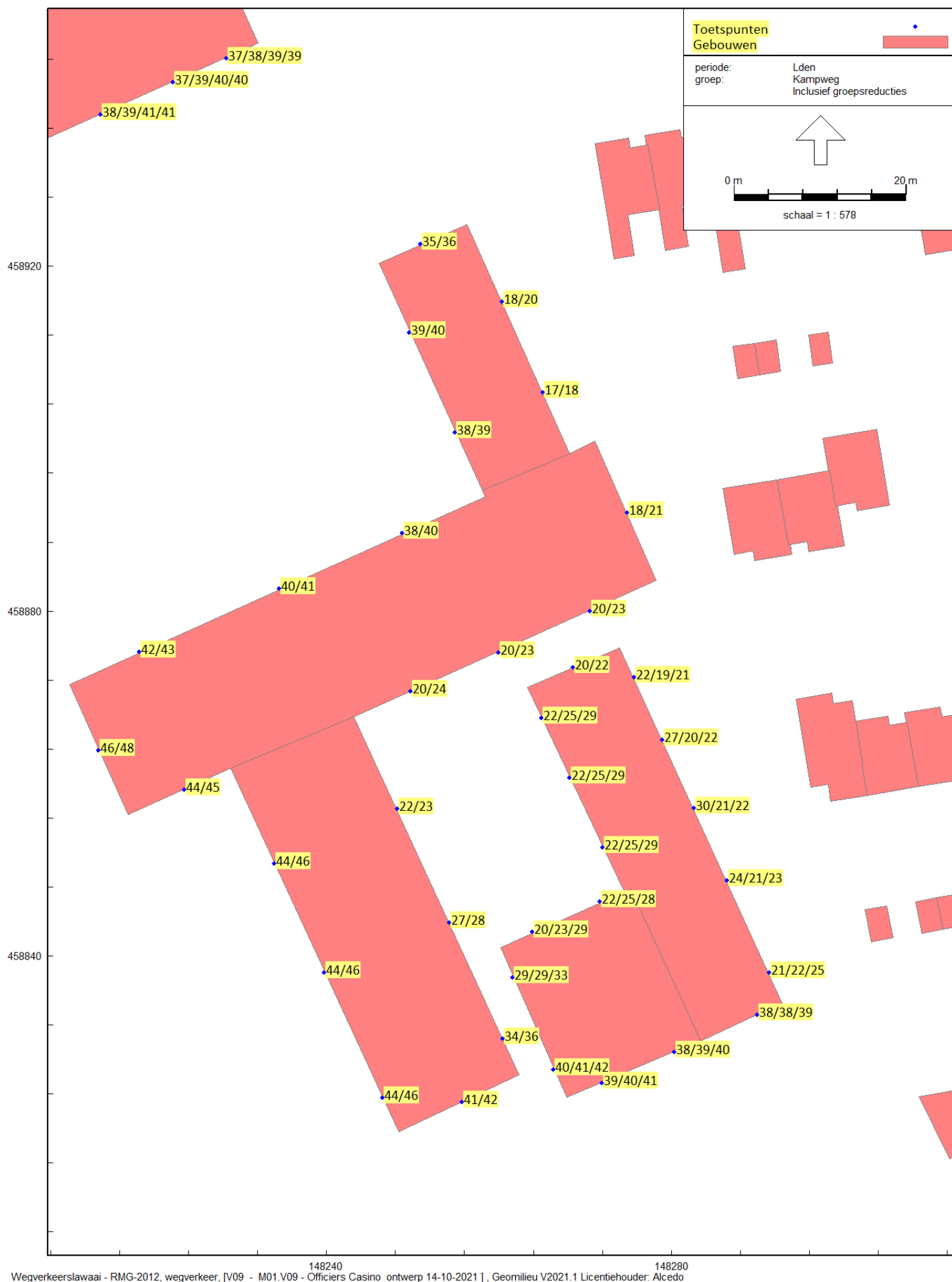
Figuur 5 Gebouw B en C: Geluidsbelastingen vanwege wegverkeer op de Kampweg inclusief 5 dB correctie conform artikel 110g Wgh Beoordelingshoogte 1,5 / 4,5 en 7,5 meter
