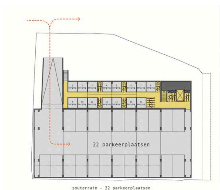
Figuur 7: Toekomstige situatie plangebied (parkeerkelder).
