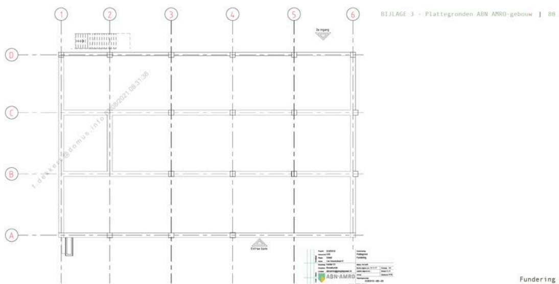
Figuur 5: Funderingstekening huidige bebouwing.
