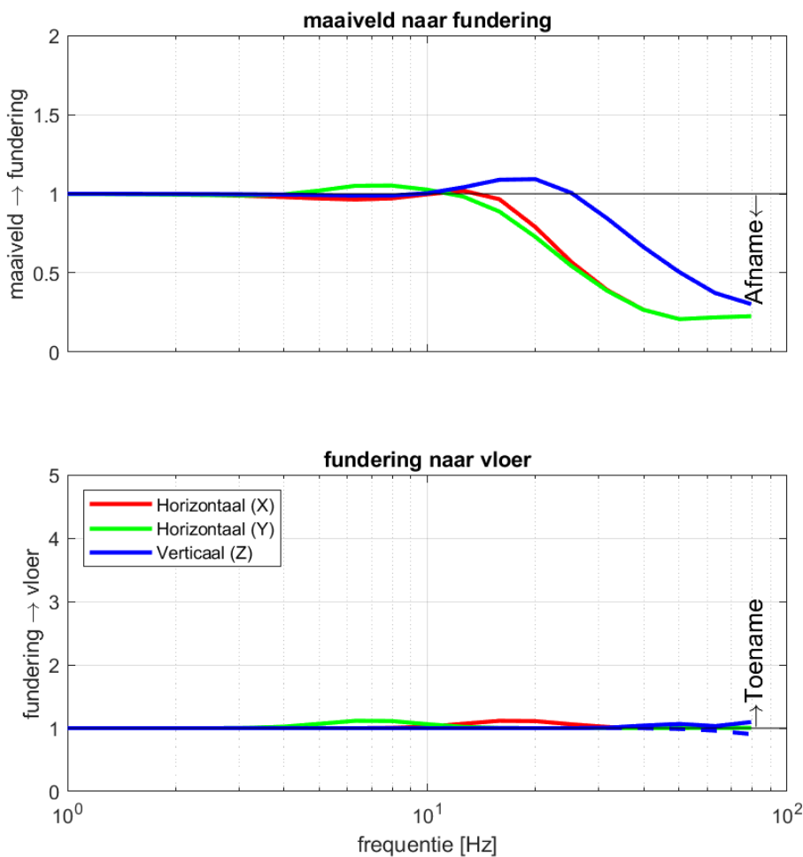
Figuur 17 Overdracht C_f (boven) en C_v van fundering naar midden vloer
