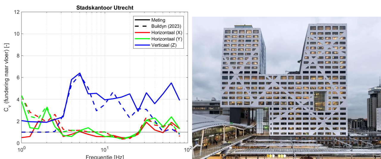
Figuur 12 Staskantoor in Utrecht, links de gemeten en berekende overdrachten, rechts een foto van het gebouw
