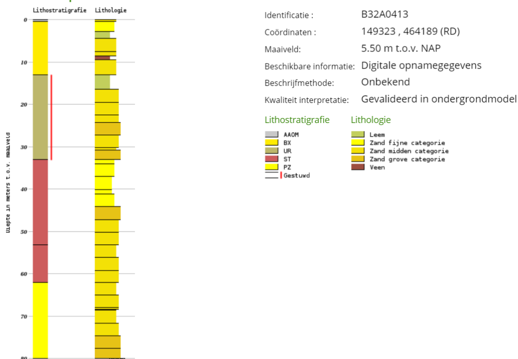
Figuur 7 Boring in het onderzoeksgebied
