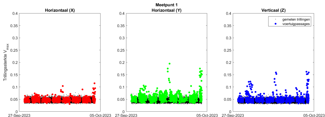
Figuur 6 Gemeten trillingen aan fundering bestaande opstal, meetpunt 1
