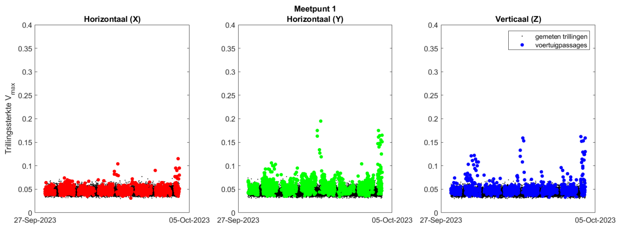
Figuur 18 Gemeten trillingen bij meetpunt 1 (fundering bestaande opstal)
