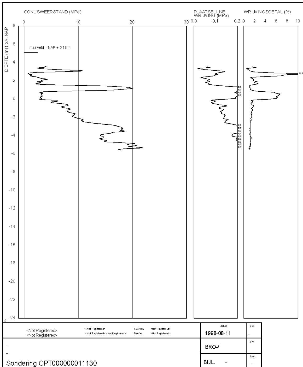
Figuur 8 Sondering nabij het onderzoeksgebied
