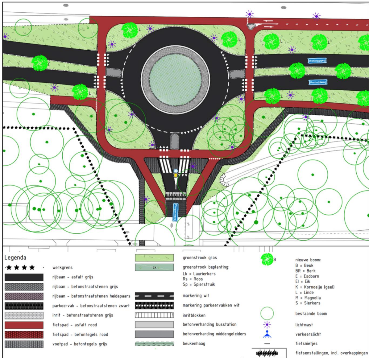
Figuur 4.2: Ontwerp rotonde (Bron: Megaborn)
