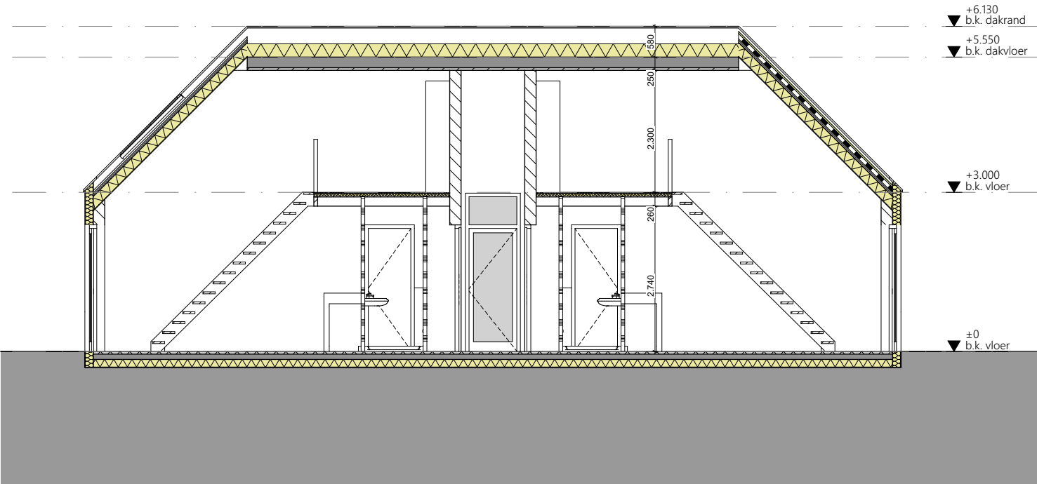
doorsnede A-A
