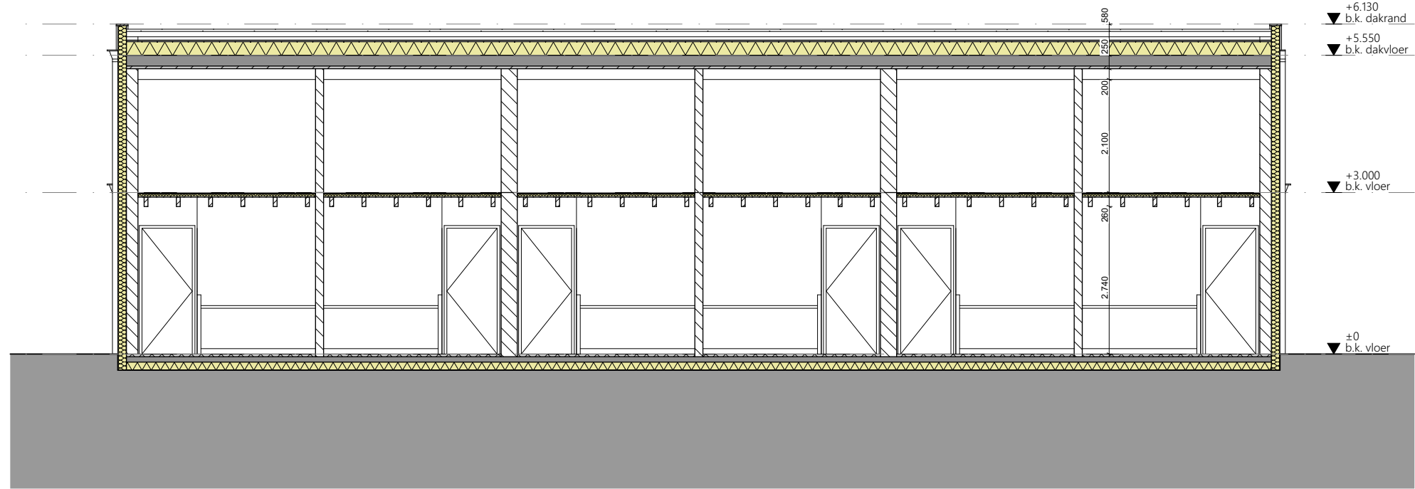
doorsnede B-B
