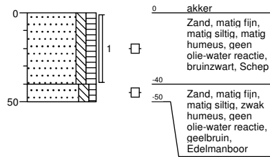
Boring: 01 boormeester J. Postma Sleuflengte [m]: 0,30 Sleufbreedte [m]: 0,30
