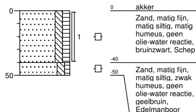
Boring: 04 boormeester J. Postma Sleuflengte [m]: 0,30 Sleufbreedte [m]: 0,30
