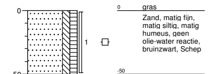
Boring: 06 boormeester J. Postma Sleuflengte [m]: 0,30 Sleufbreedte [m]: 0,30
