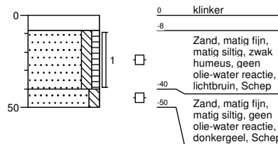
Boring: 05 boormeester J. Postma Sleuflengte [m]: 0,30 Sleufbreedte [m]: 0,30
