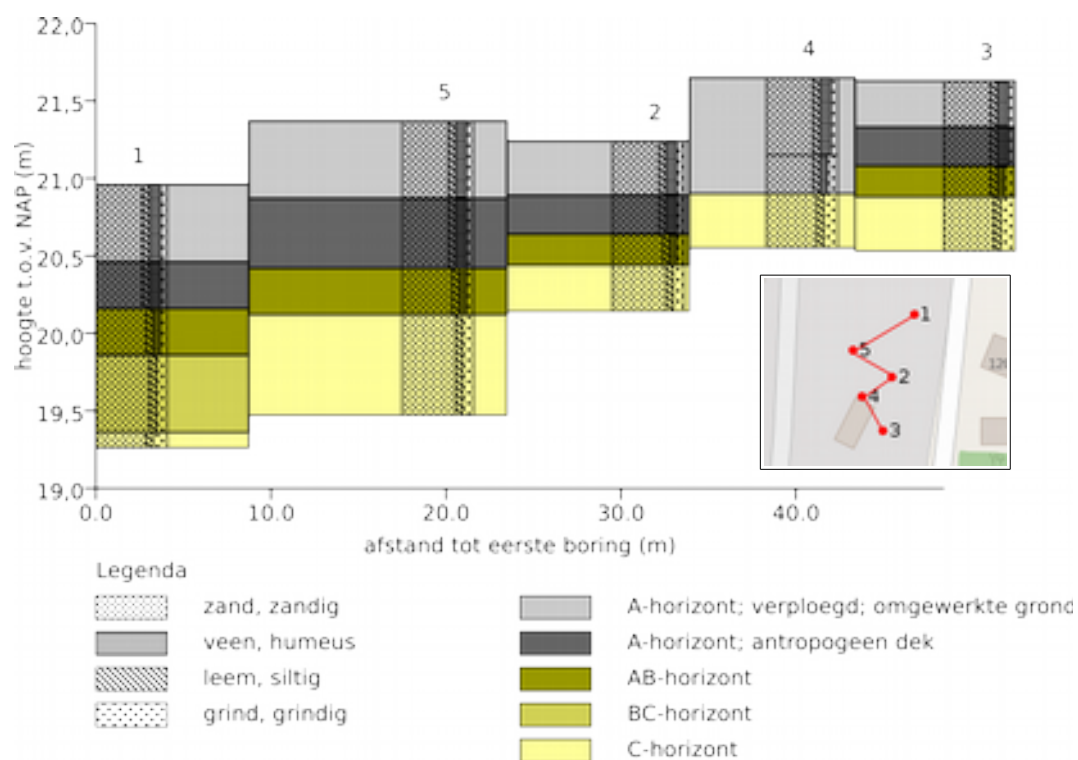
Figuur 18: Schematische doorsnede.
