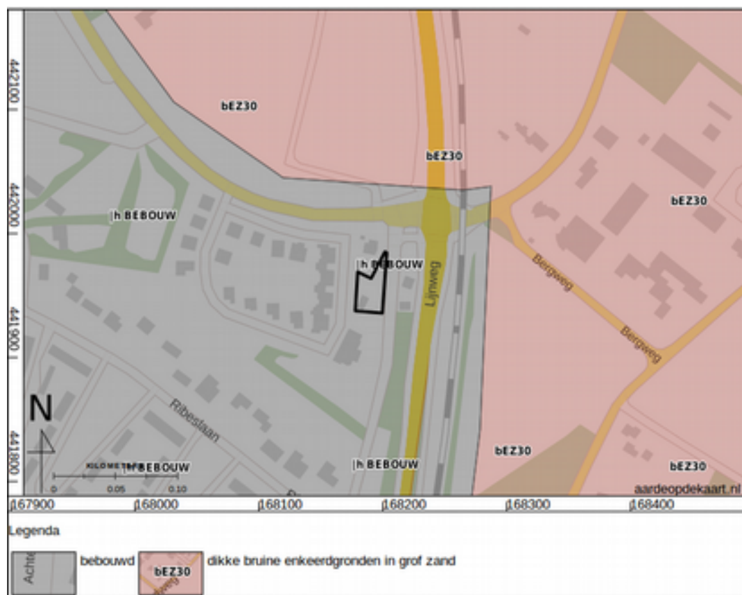
Figuur 4: Bodemkaart.
