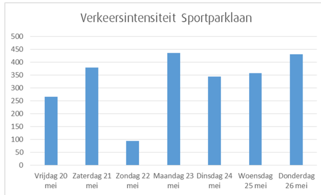
Figuur 3.4: Verkeersintensiteiten Sportparklaan, motorvoertuigen per etmaal gedurende de telperiode
