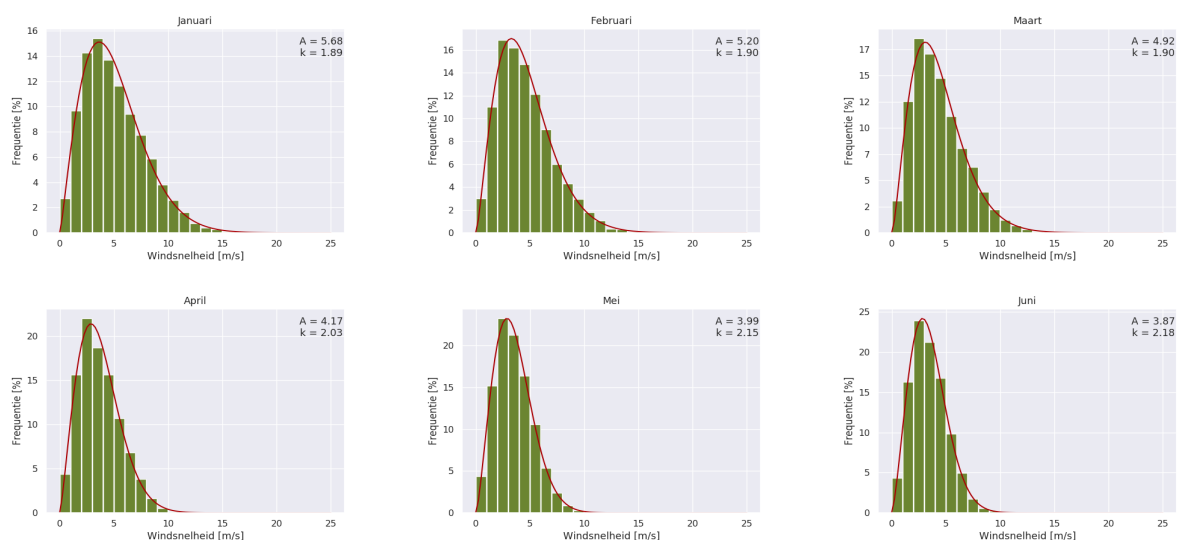
Figuur 2.6: Maandelijks frequentie-verdeling met Weibull-verdeling
