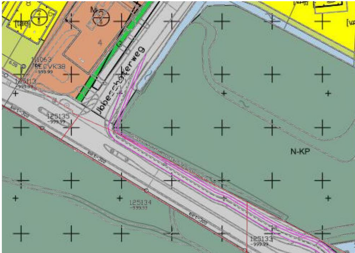
Afbeelding 1.1 Verbreding fietspad
