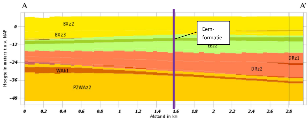
Afbeelding 3.3 Verticale doorsnede REGIS II
