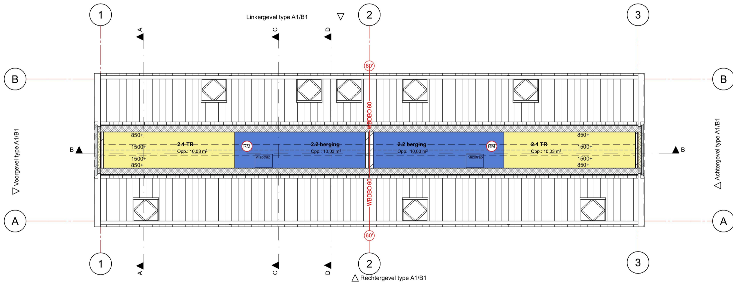
Begane grond
