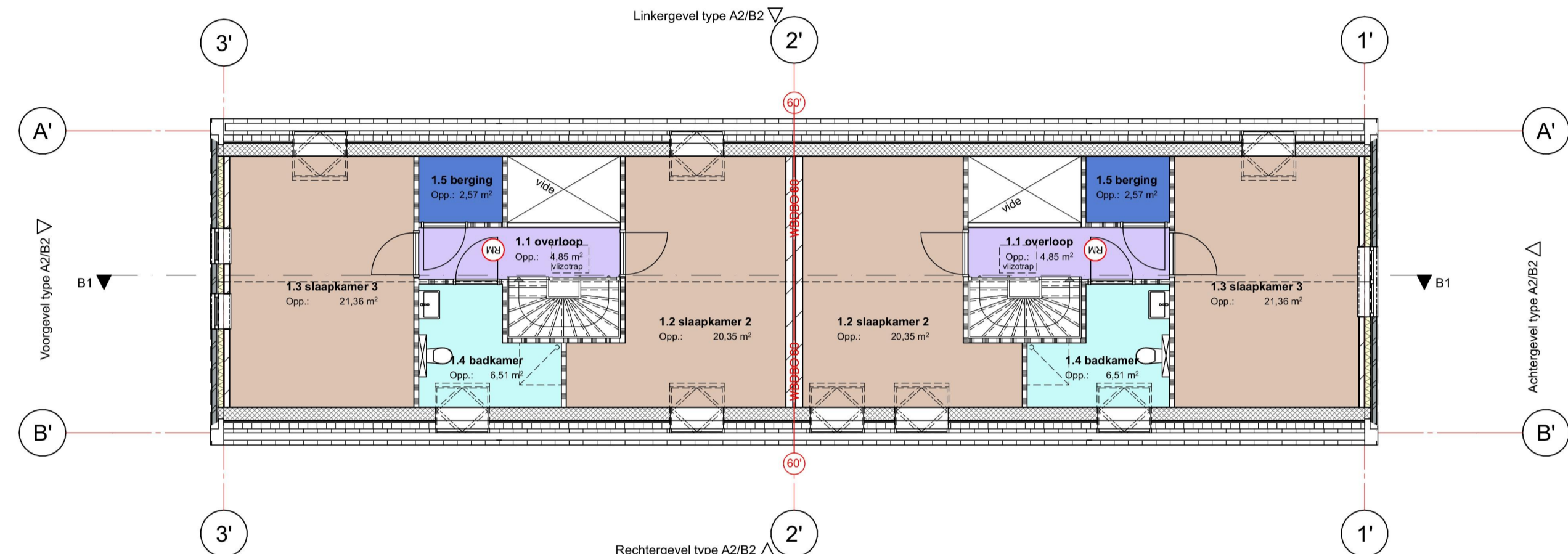
1e verdieping
