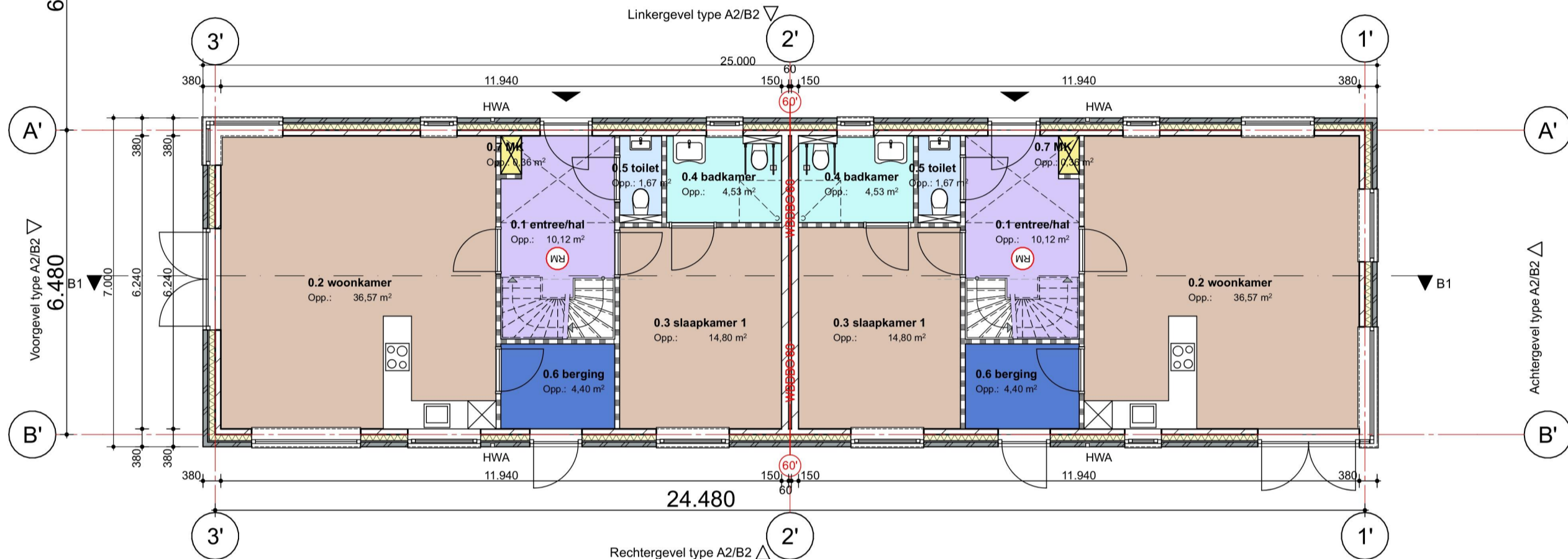
Begane grond
