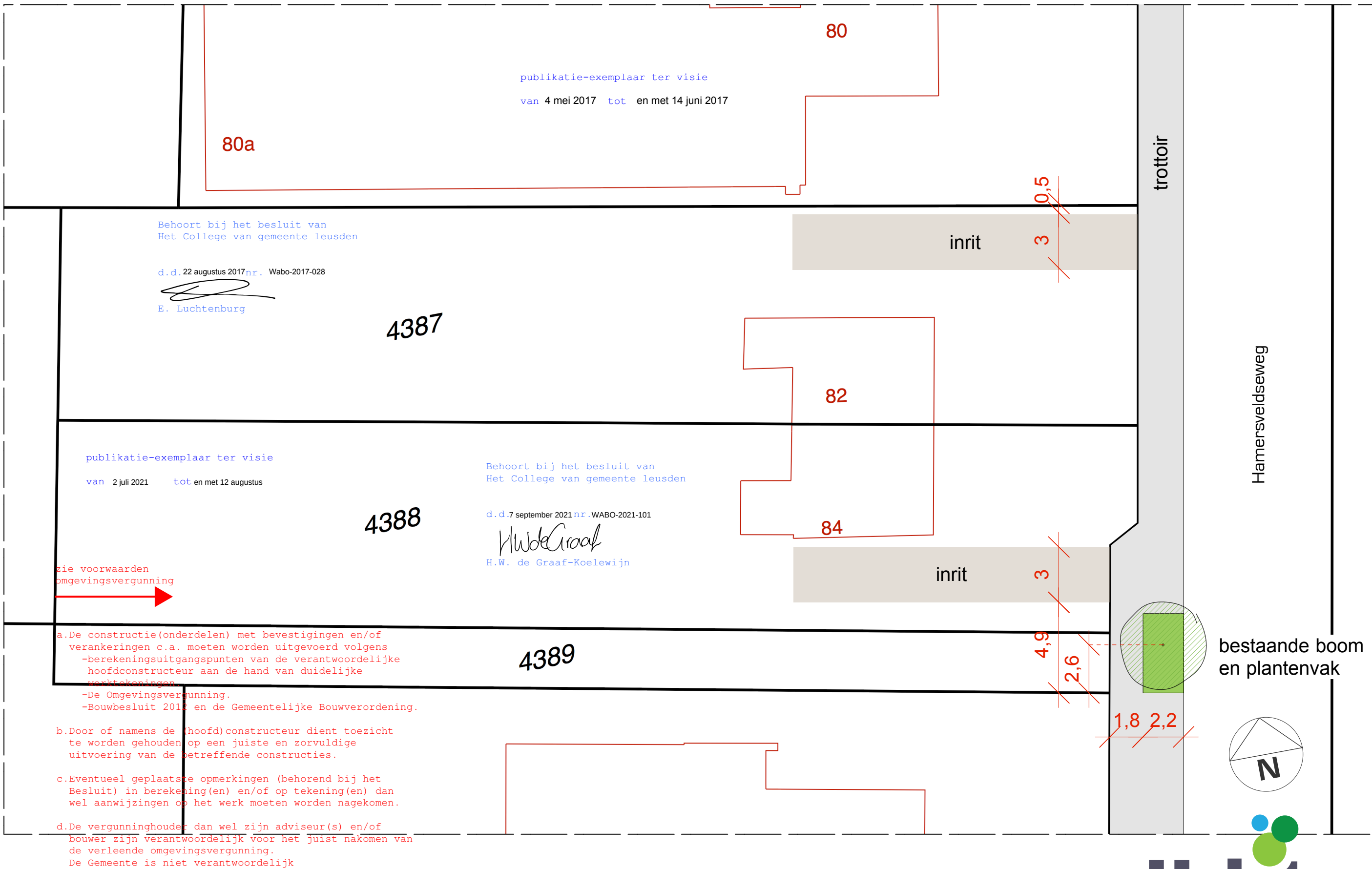
SITUATIE - HAMERSVELDSEWEG BESTAAND kavel 4387, 4388 en 4389 d.d. 20 02 2017 schaal 1:200
