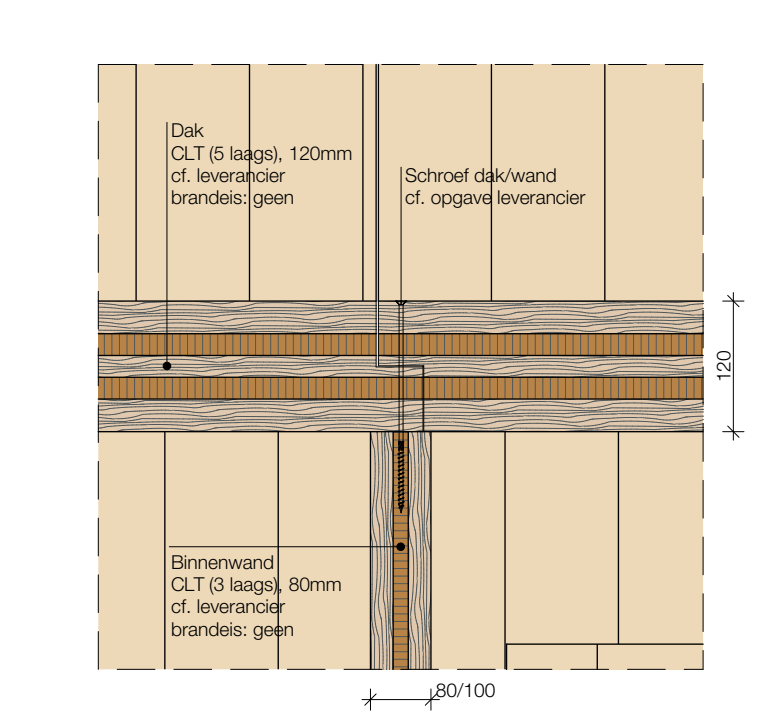
V.08 Aansluiting dak/binnenwand 1:10
