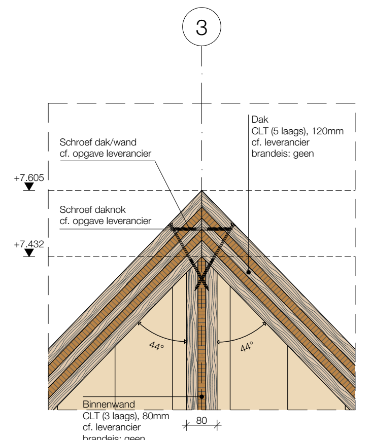
V.04 Aansluiting daknok 1:10
