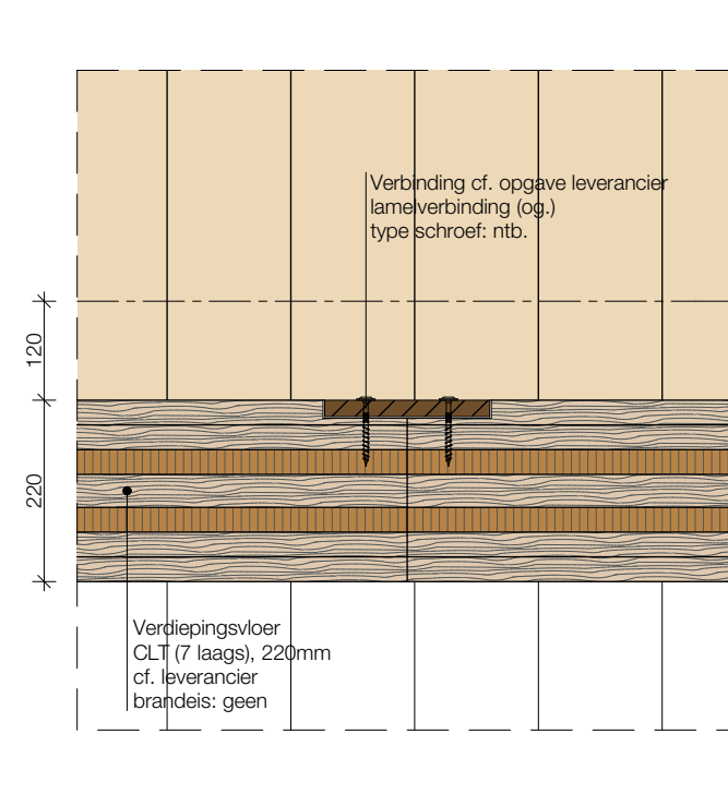
V.06 Aansluiting vloer/vloer 1:10
