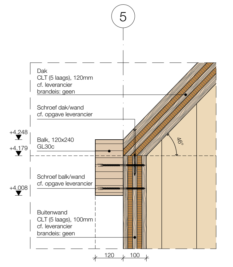
V.03 Aansluiting buitenwand/dak 1:10
