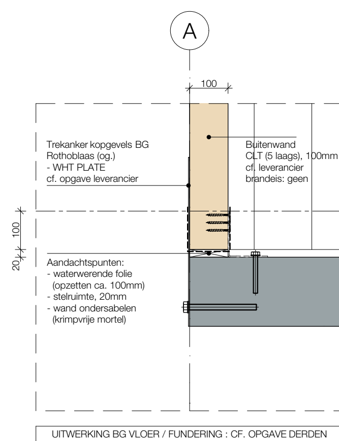
V.01b Aansluiting dwarswand/BG vloer 1:10
