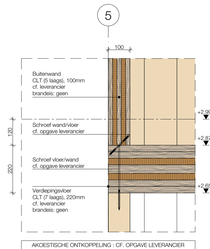
V.02 Aansluiting buitenwand/vloer 1:10
