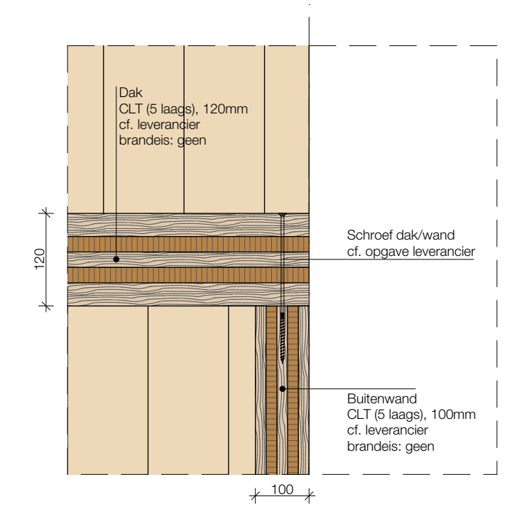
V.09 Aansluiting dak/buitenwand 1:10
