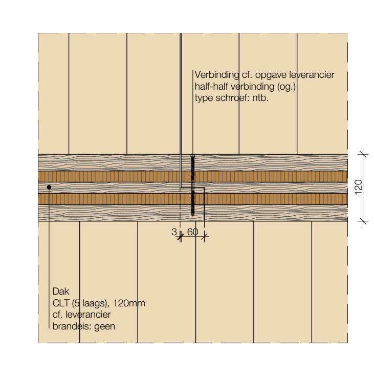
V.07 Aansluiting dak/dak 1:10
