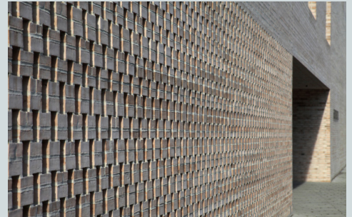
Verfijning in de plint, bijvoorbeeld in (deels) opengewerkt metselwerk; Stadtbibliothek Heidenheim (Max Dudler)
