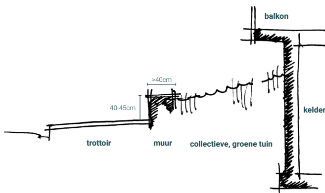
Principe-doorsnede trottoir, tuin en tuinmuur
