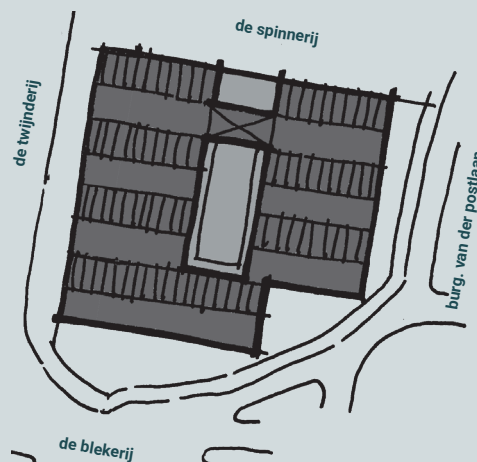
Bovenaanzicht mogelijk bouwvolume met verplichte nokrichting
