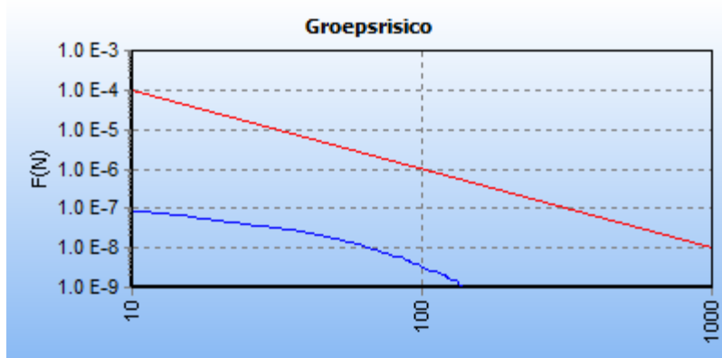
11.1 Figuur 5.1 FN curve voor 3416_leiding-A-510-deel-1 van N.V. Nederlandse Gasunie voor de kilometer tussen stationing 1540.00 en stationing 2540.00
