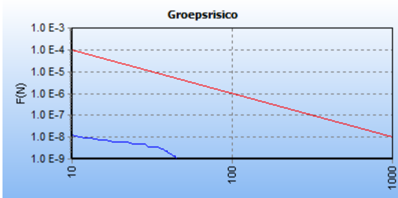
5.1 Figuur 5.1 FN curve voor 3416_leiding-A-510-deel-1 van N.V. Nederlandse Gasunie voor de kilometer tussen stationing 1490.00 en stationing 2490.00
