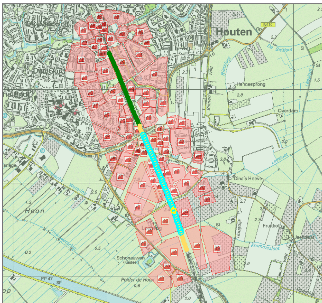
Figuur 4. Kilometer hoogste groepsrisico, transport ontwerp Basisnet Spoor, gridgrootte is 1000 m
