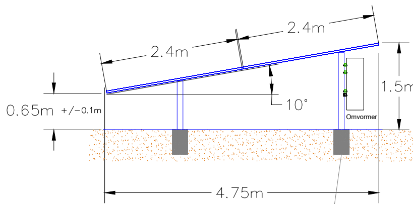
Betonfundering (volgens de definitieve bodemanalyse)
