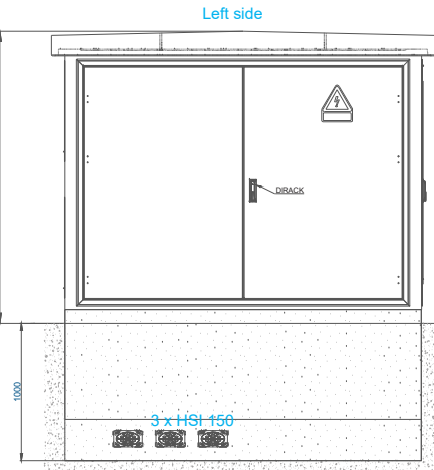
Betonfundering (volgens de definitieve bodemanalyse)
