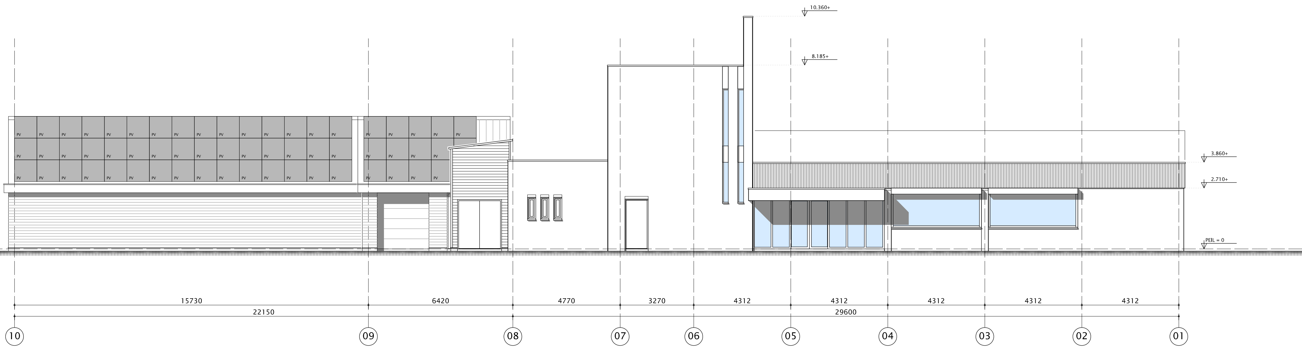
VOORGEVEL
