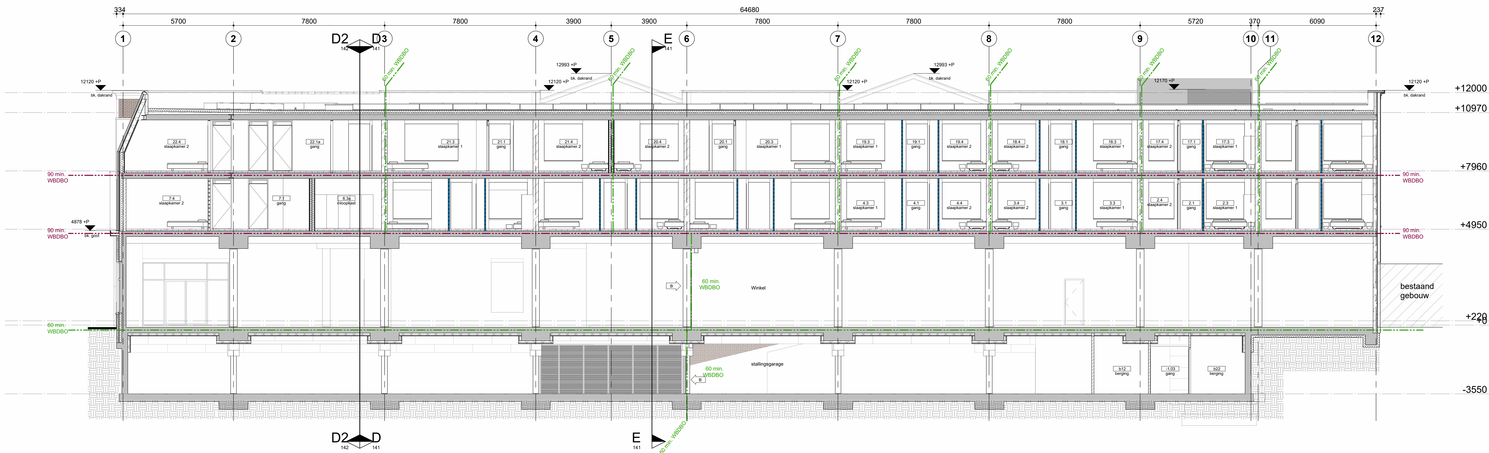
doorsnede A-A
