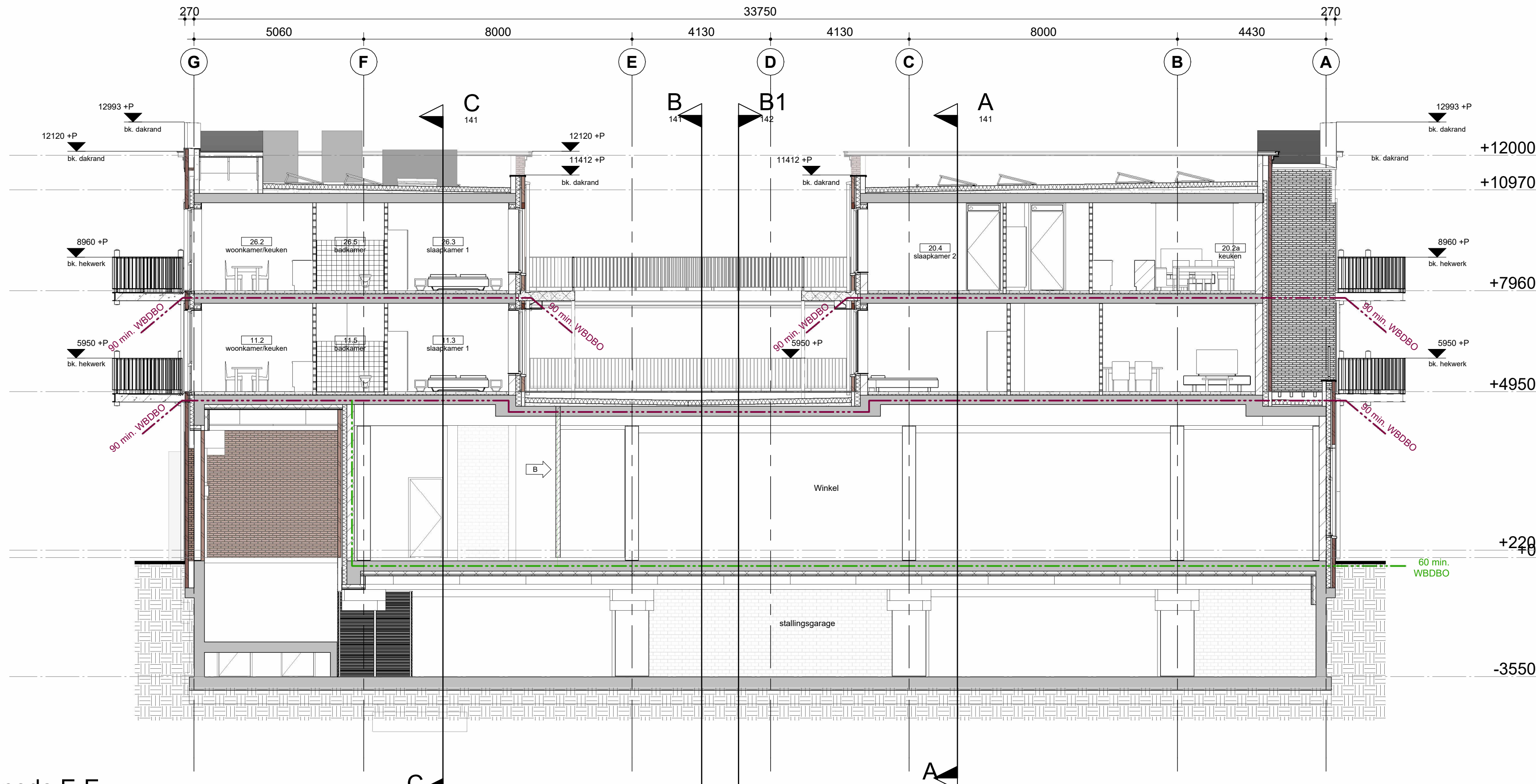
doorsnede E-E
