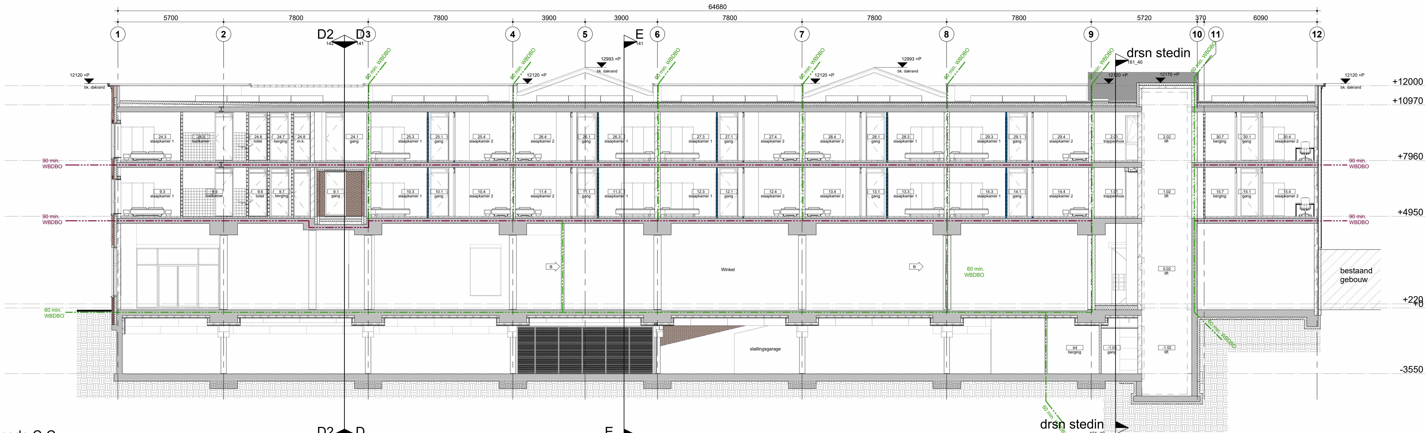
doorsnede C-C
