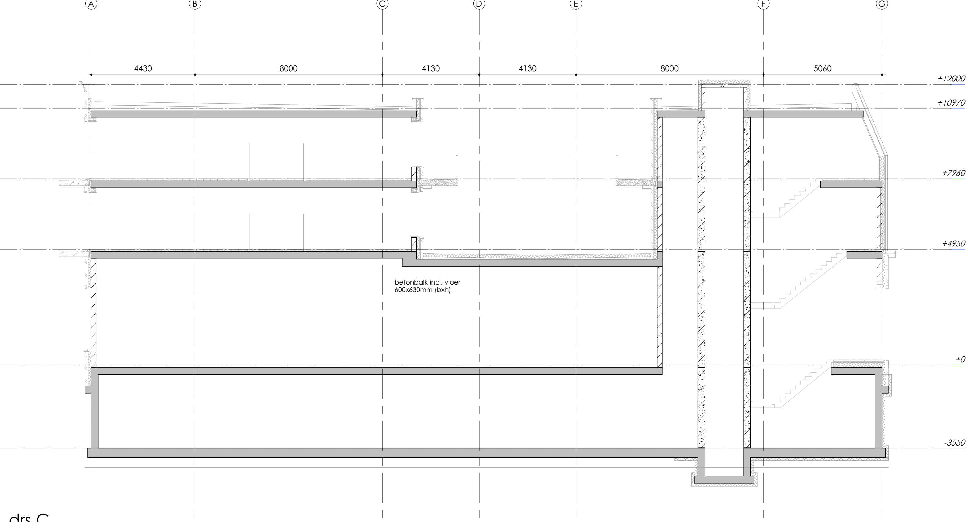
drs C 1 : 100
