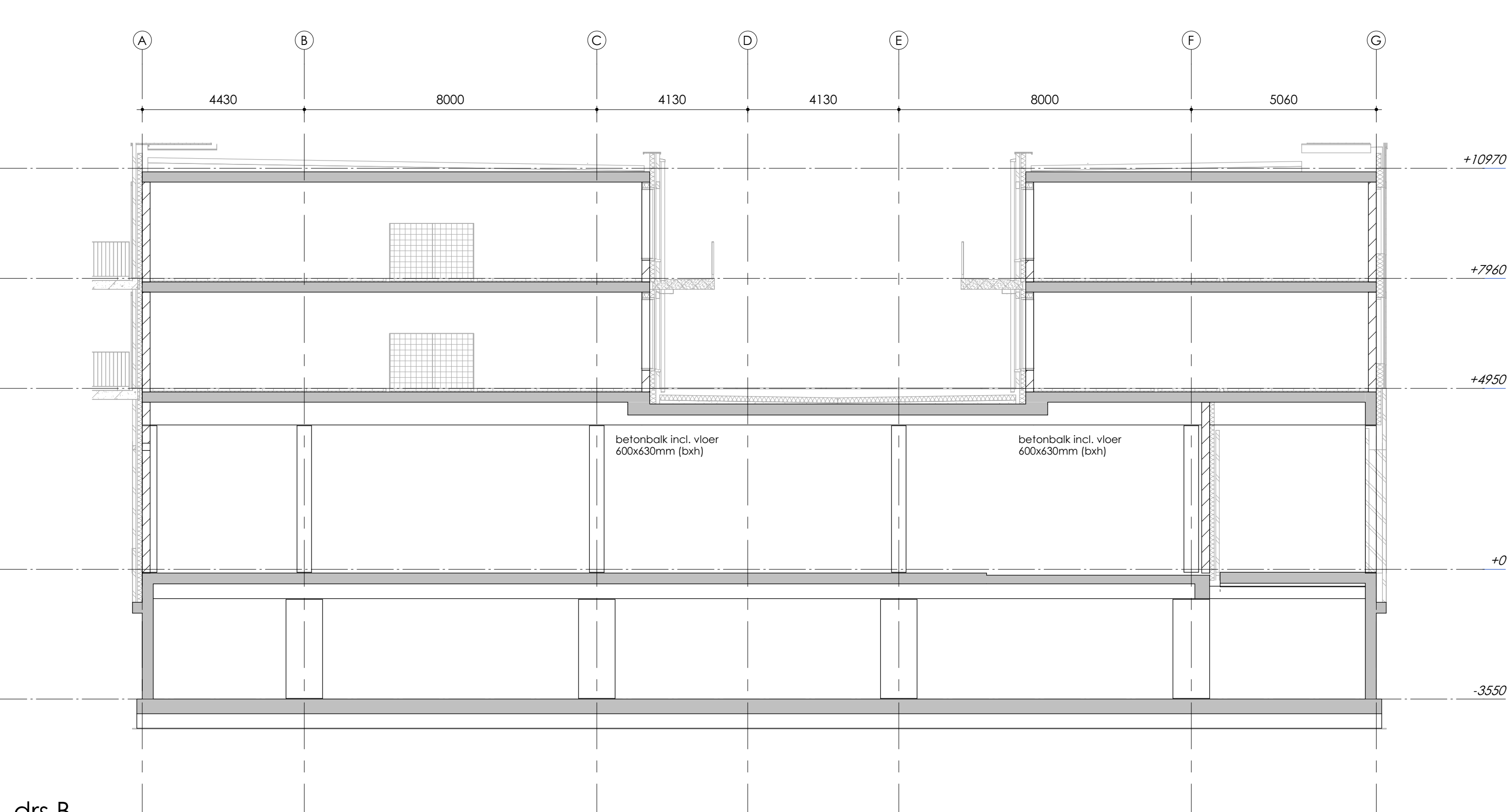
drs B 1 : 100
