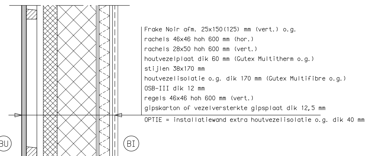
DETAIL C2b buitengevel
