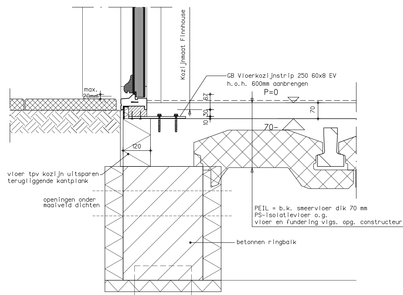
DETAIL C1b onderdorpel voordeur
