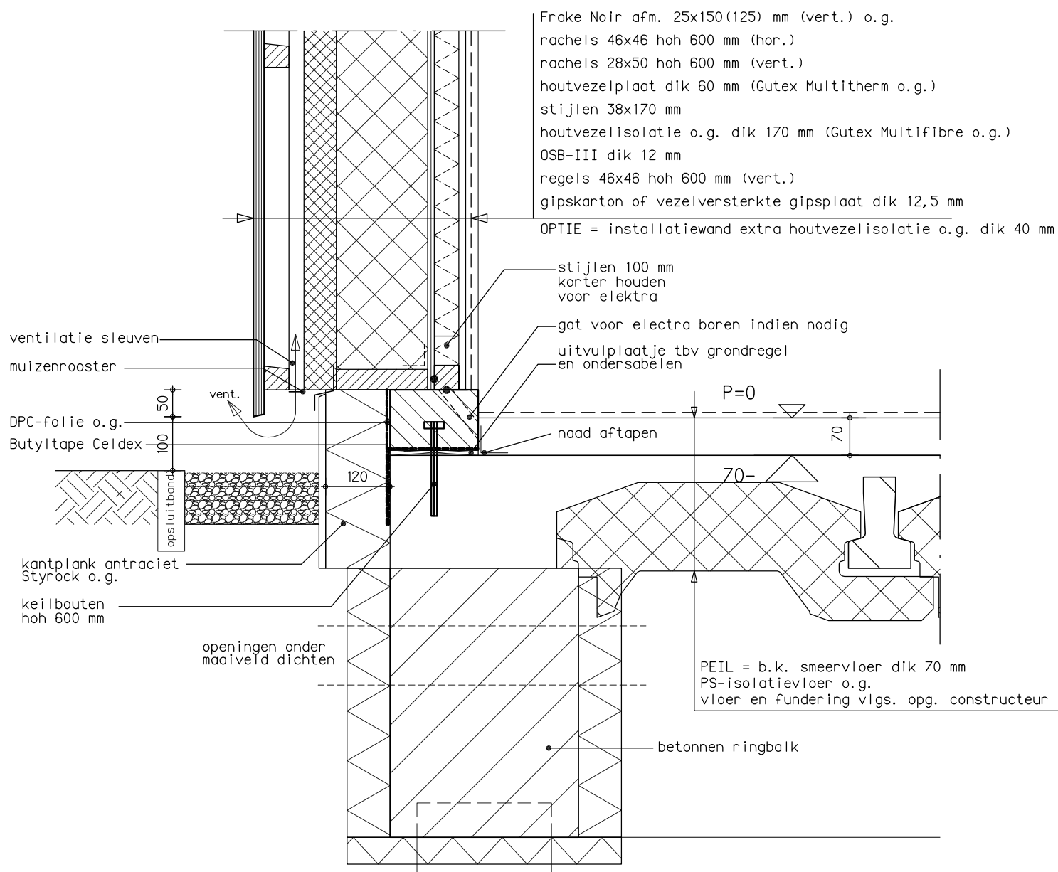
DETAIL C1a funderingsdetail gevels hout verticale delen
