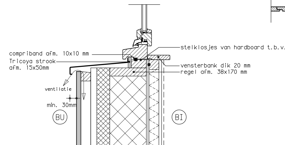
DETAIL C3a buitenkozijn hout HSB
