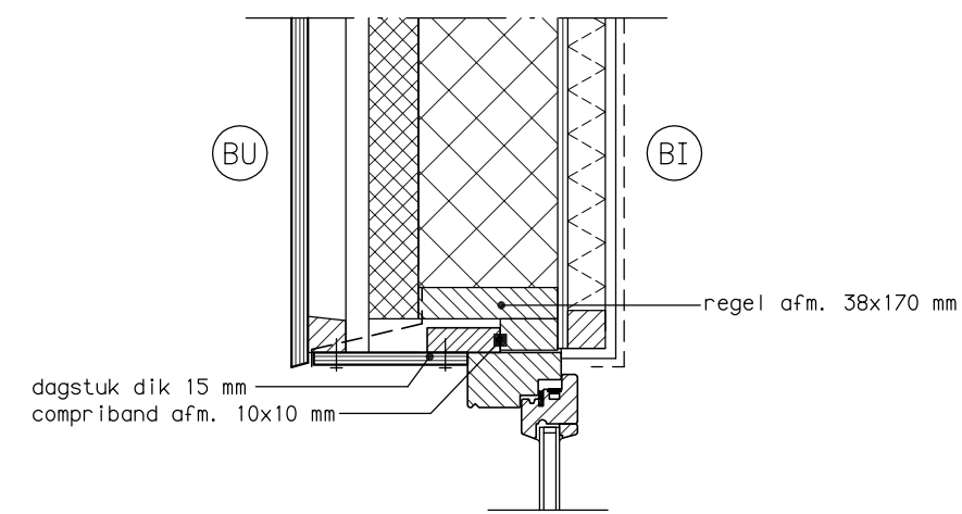
DETAIL C3a buitenkozijn hout HSB
