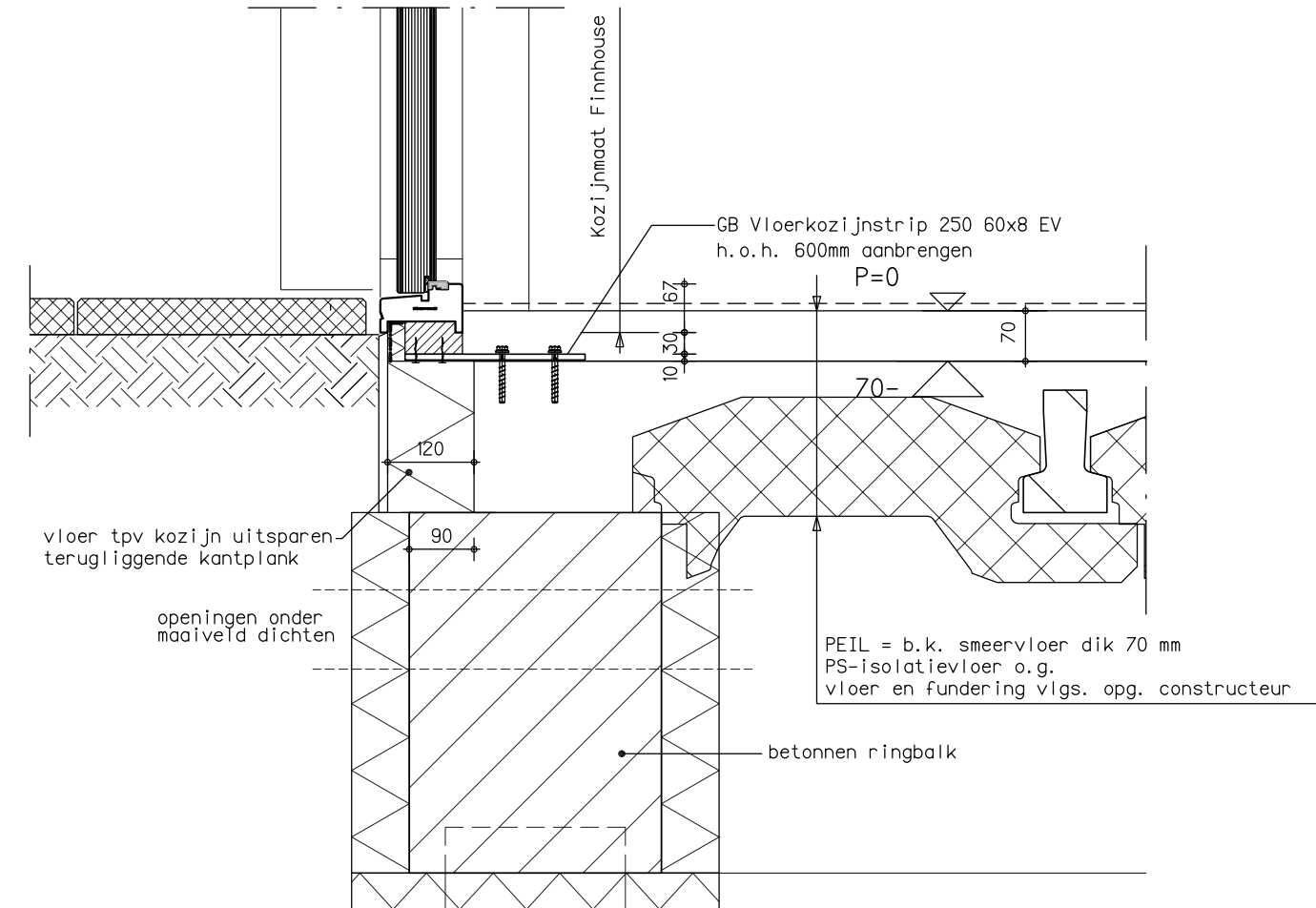
DETAIL C1d onderdorpel naar buiten draaiende deur
