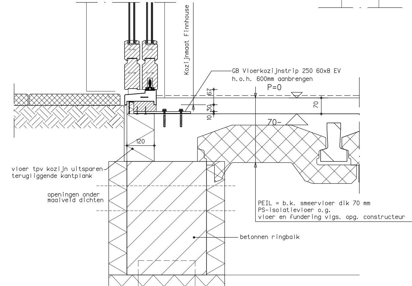
DETAIL C1e onderdorpel schuifpui
