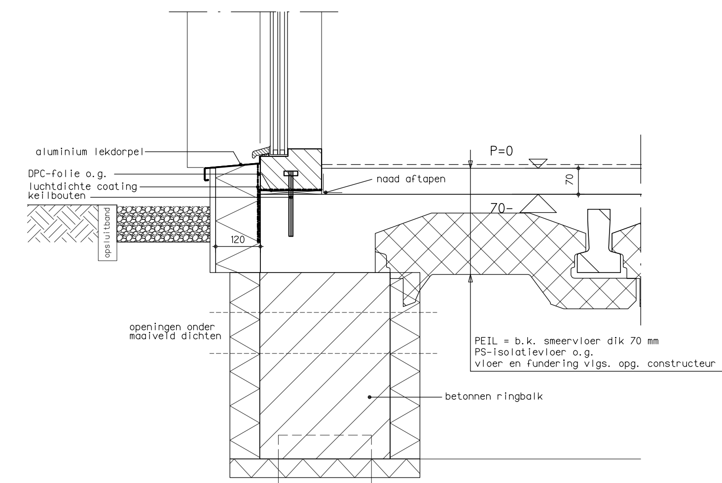
DETAIL C1c onderdorpel glaspui
