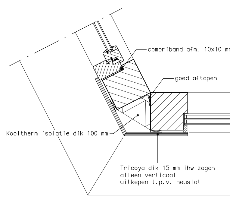
DETAIL C3c hoekoplossing glas-kozijn gl3
