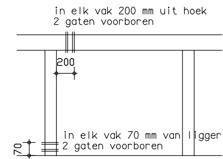
principe gaten t.b.v. elektra
