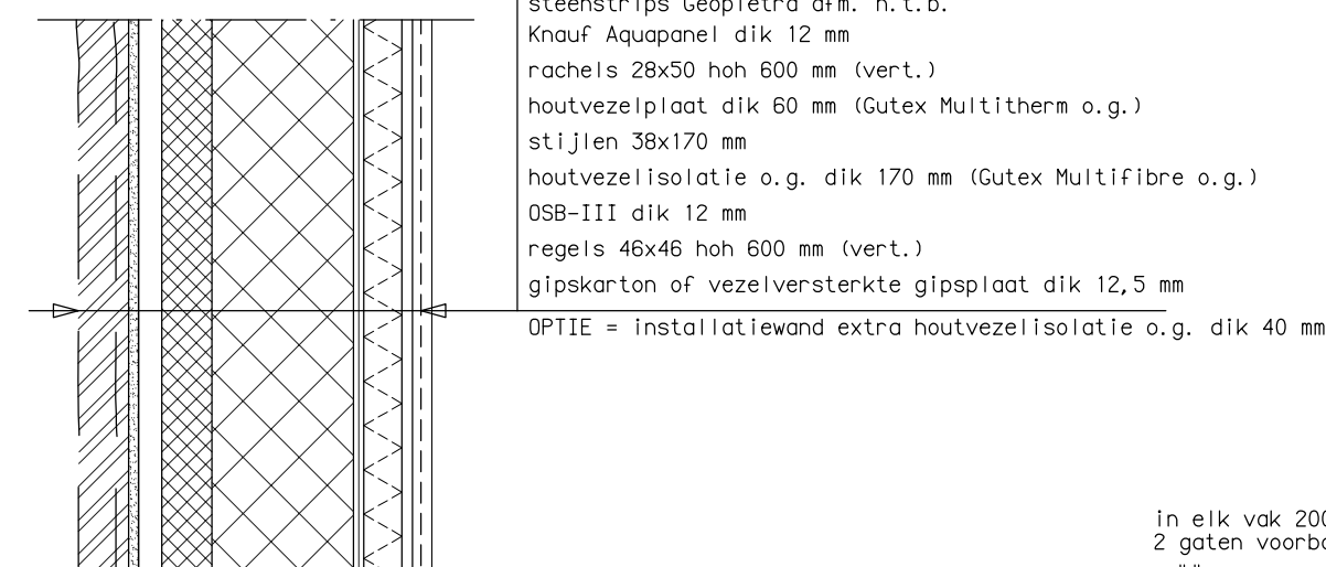
DETAIL C2c buitengevel t.p.v. steenstrips
