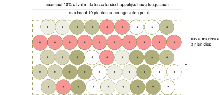
Inboet principe landschappelijke haag
