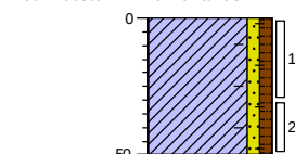
Boring: 4 Datum: 11-6-2020 Boormeester: Renze van den Brink
