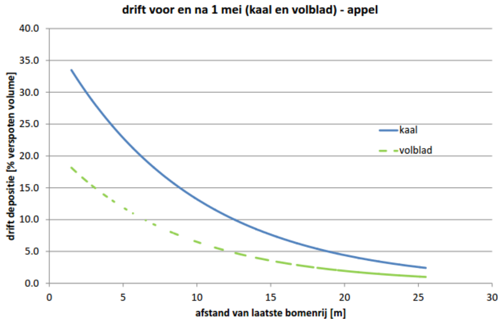
Afbeelding 4 Driftdepositie (% van de dosering) op grondoppervlak naast het perceel voor een standaard boomgaardspuit in de volblad (na 1 mei) en de kaalblad (voor 1 mei) situatie (PRI, 2015).
