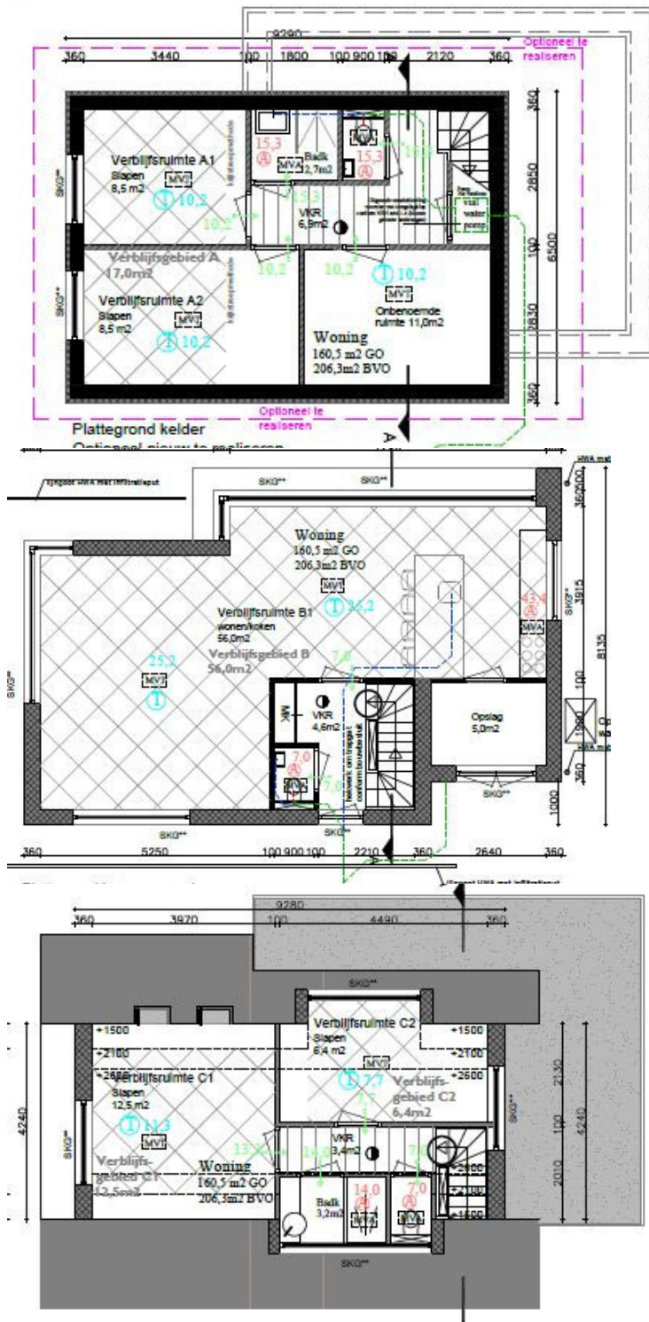
Figuur 3.5 plattegronden woning 2
