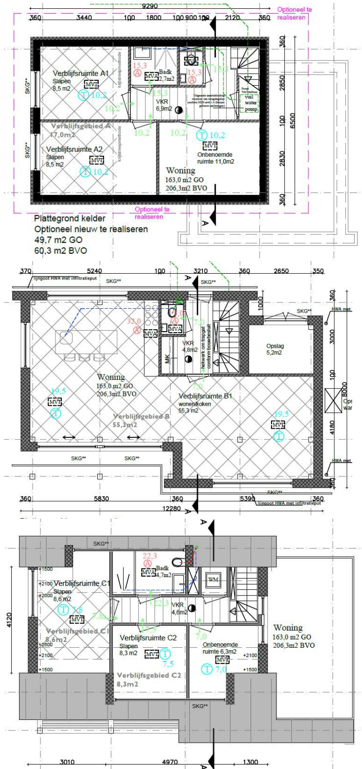
Figuur 3.4 plattegronden woning 1
