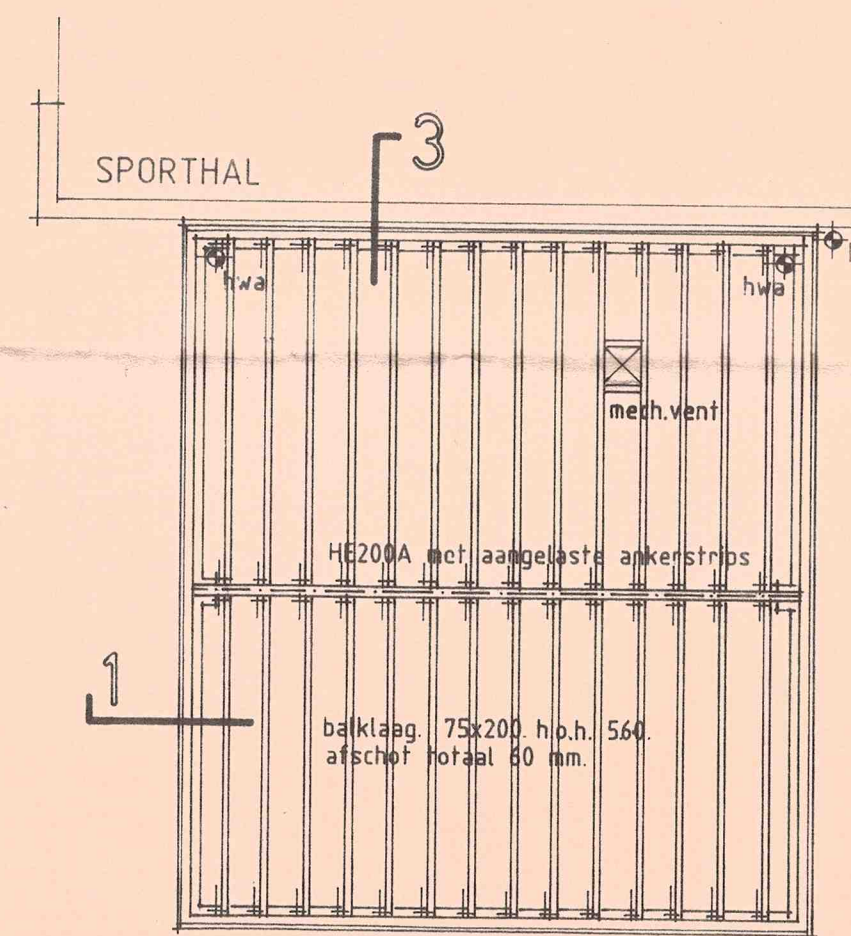
platbalklaag
