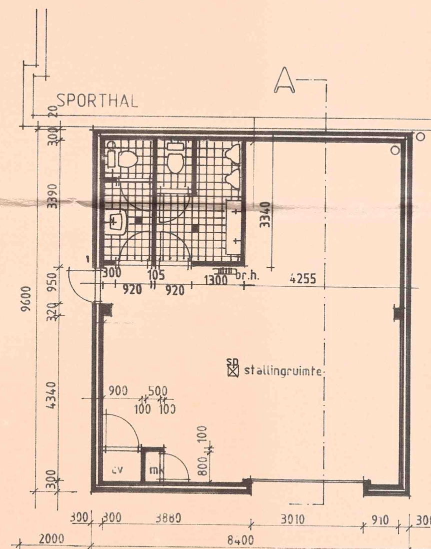
plattegrond
