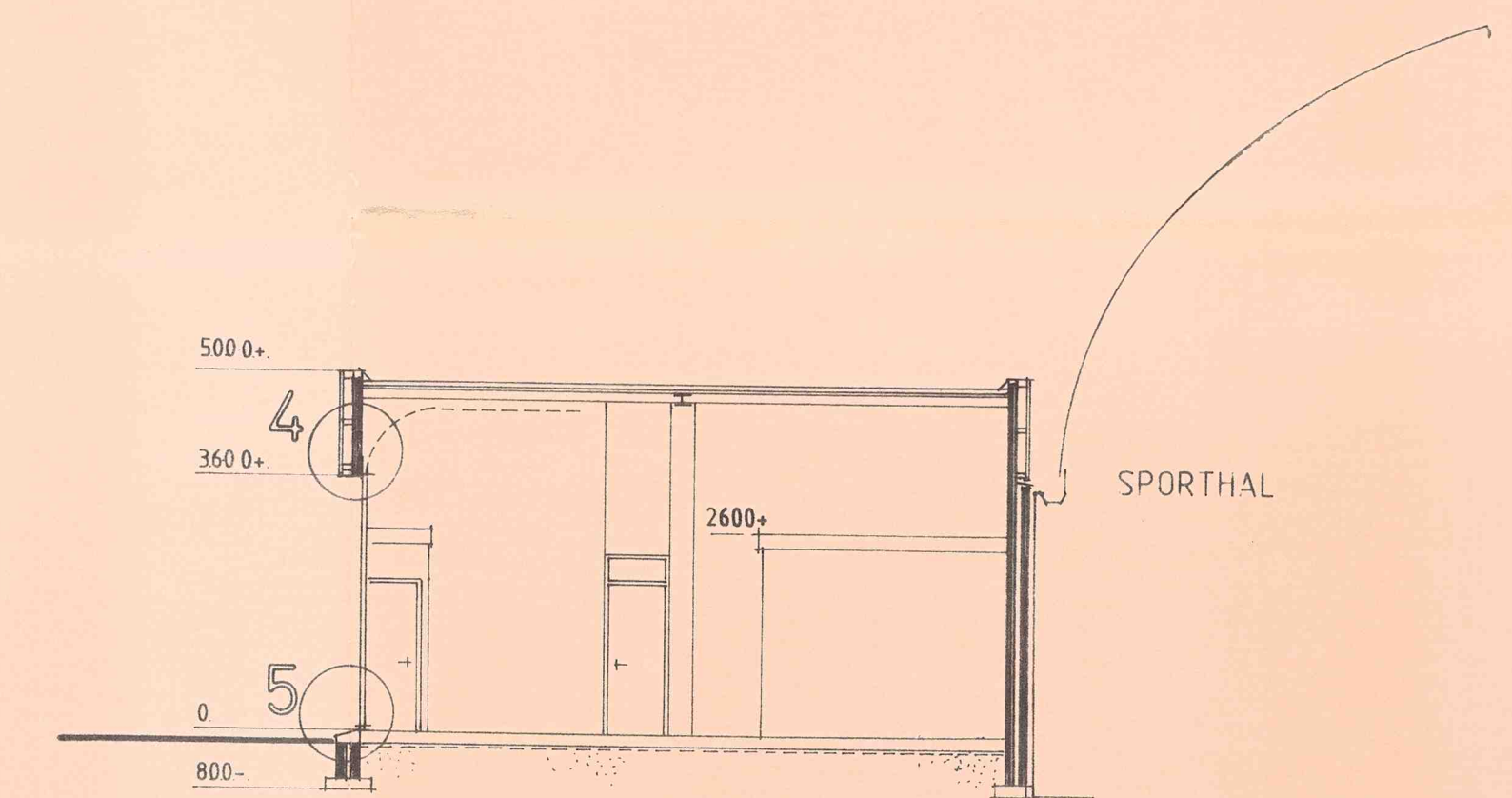
doorsnede A
