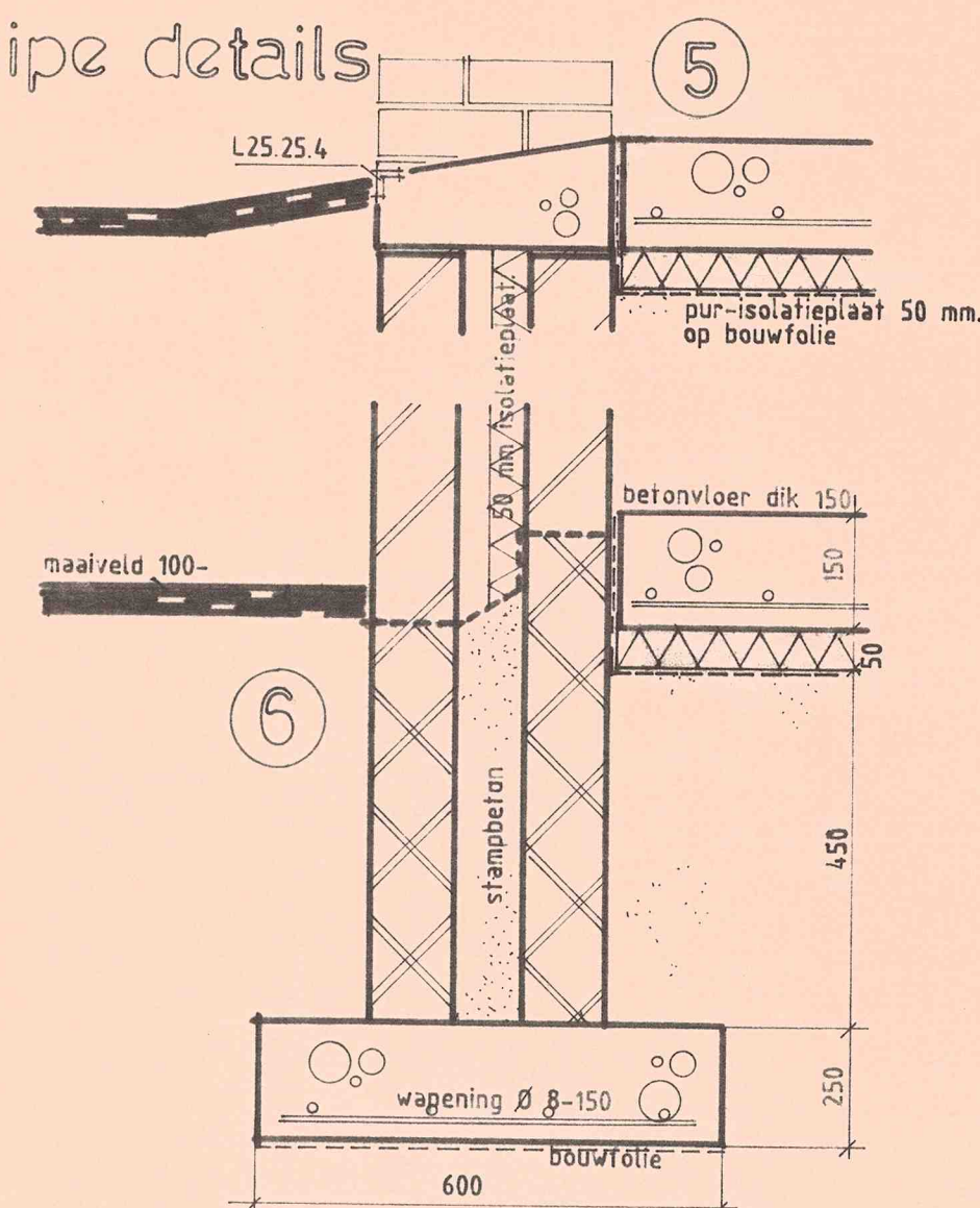
platbalklaag
