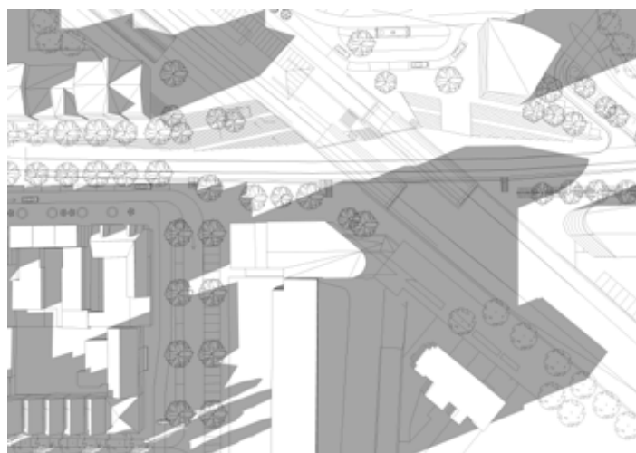
21 december 13.00 uur
