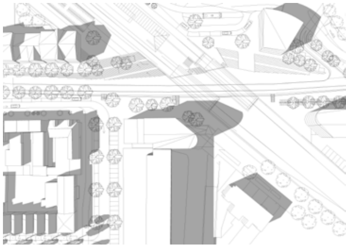
21 maart 13.00 uur
