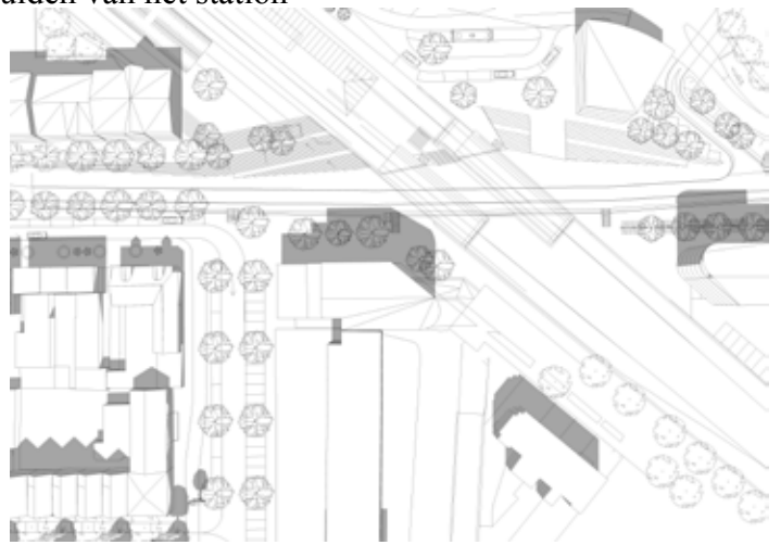
21 juni 10.00 uur
