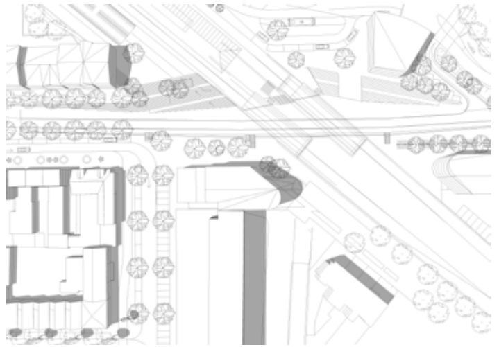
21 juni 13.00 uur
