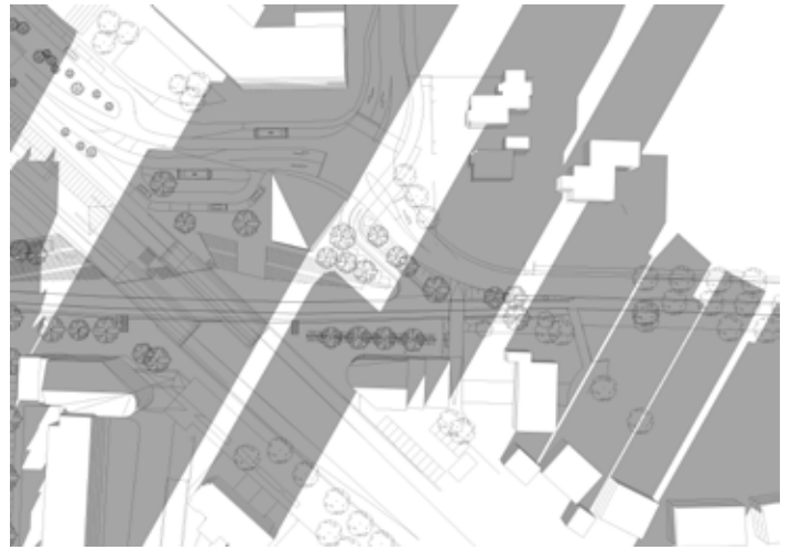
21 december 10.00 uur
