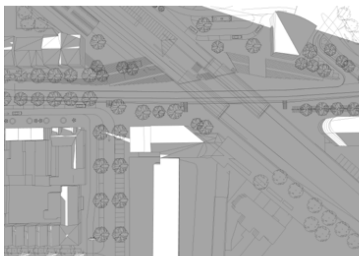
21 december 16.00 uur
