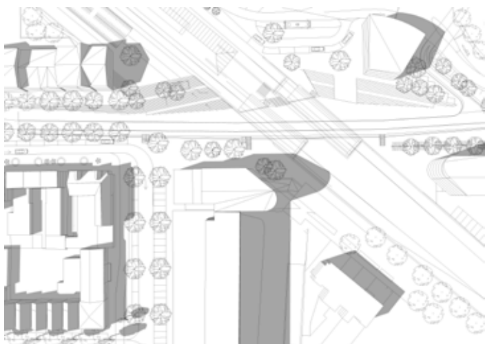
21 september 13.00 uur
