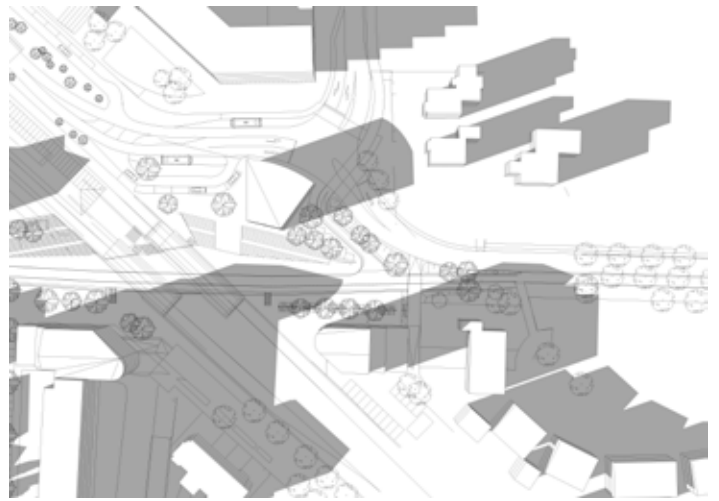
21 december 13.00 uur
