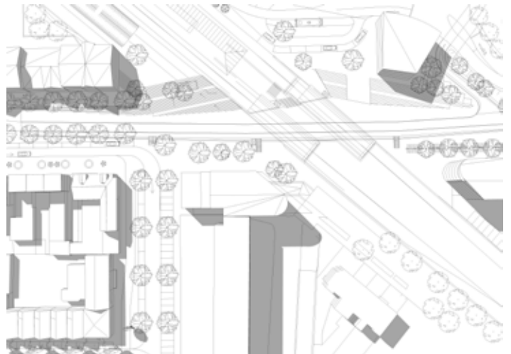
21 juni 16.00 uur
