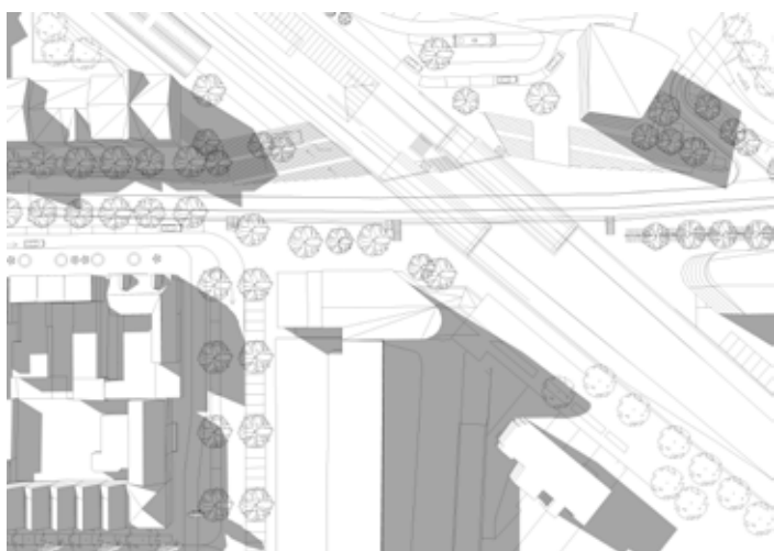
21 september 16.00 uur
