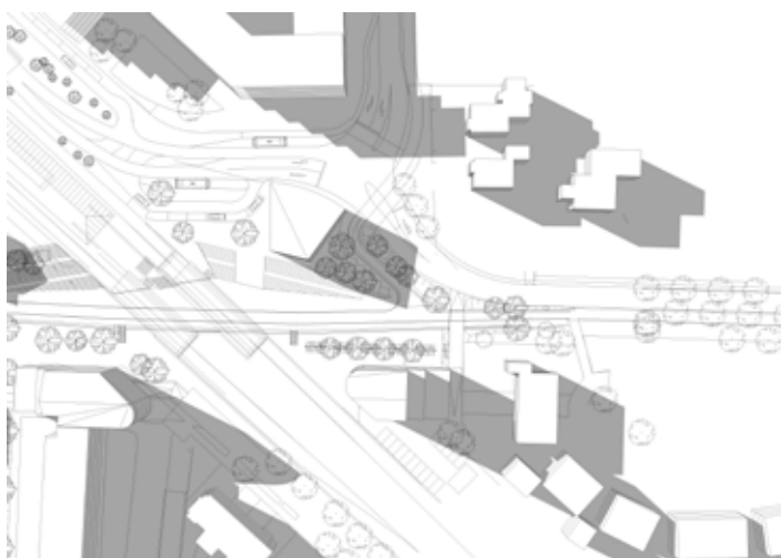
21 maart 16.00 uur
