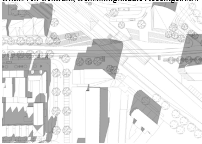
21 maart 10.00 uur
