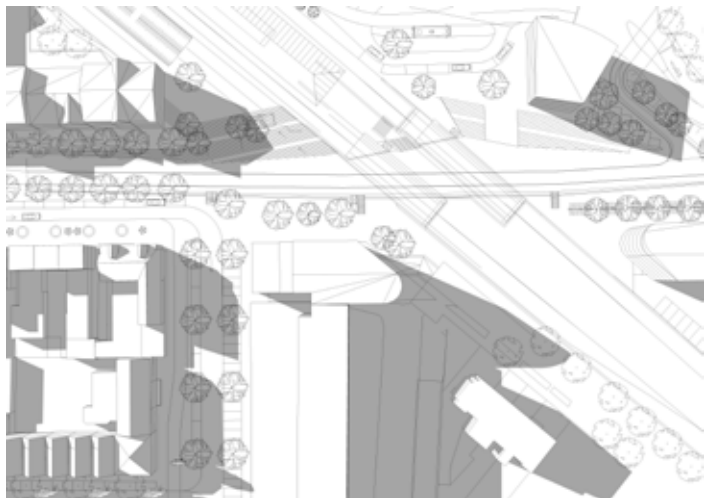
21 maart 16.00 uur
