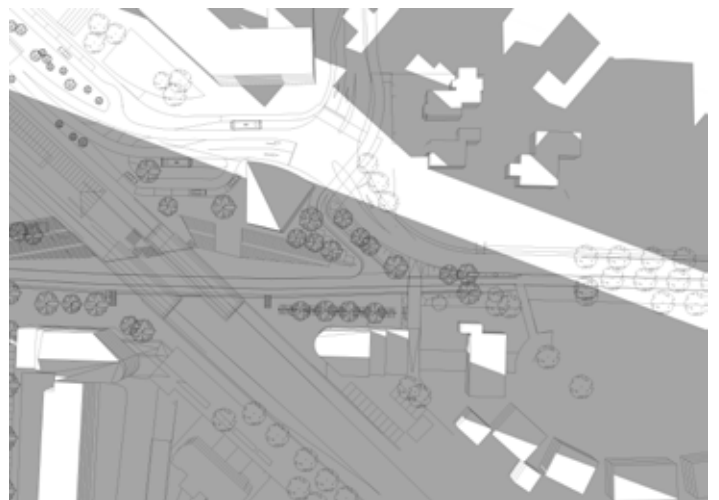
21 december 16.00 uur
