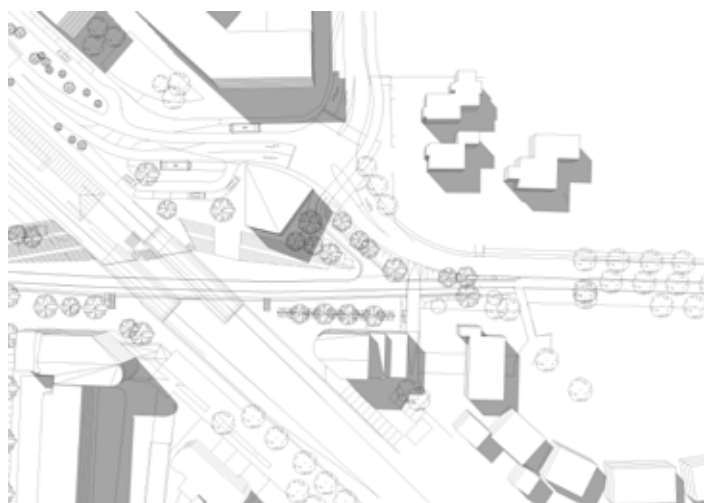
21 juni 16.00 uur
