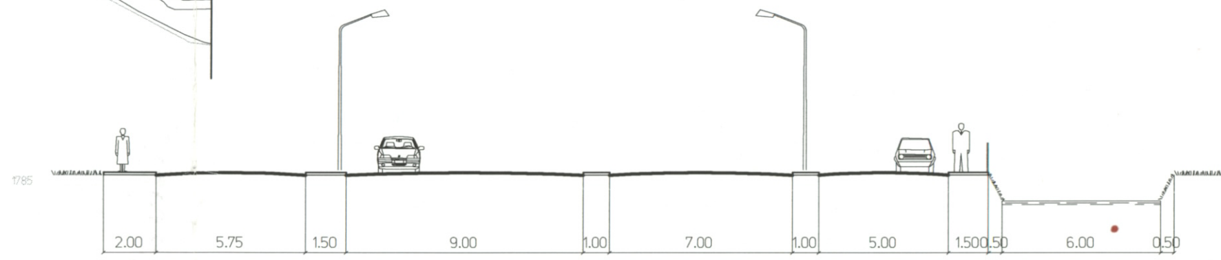
Dwarsprofiel 1:200
