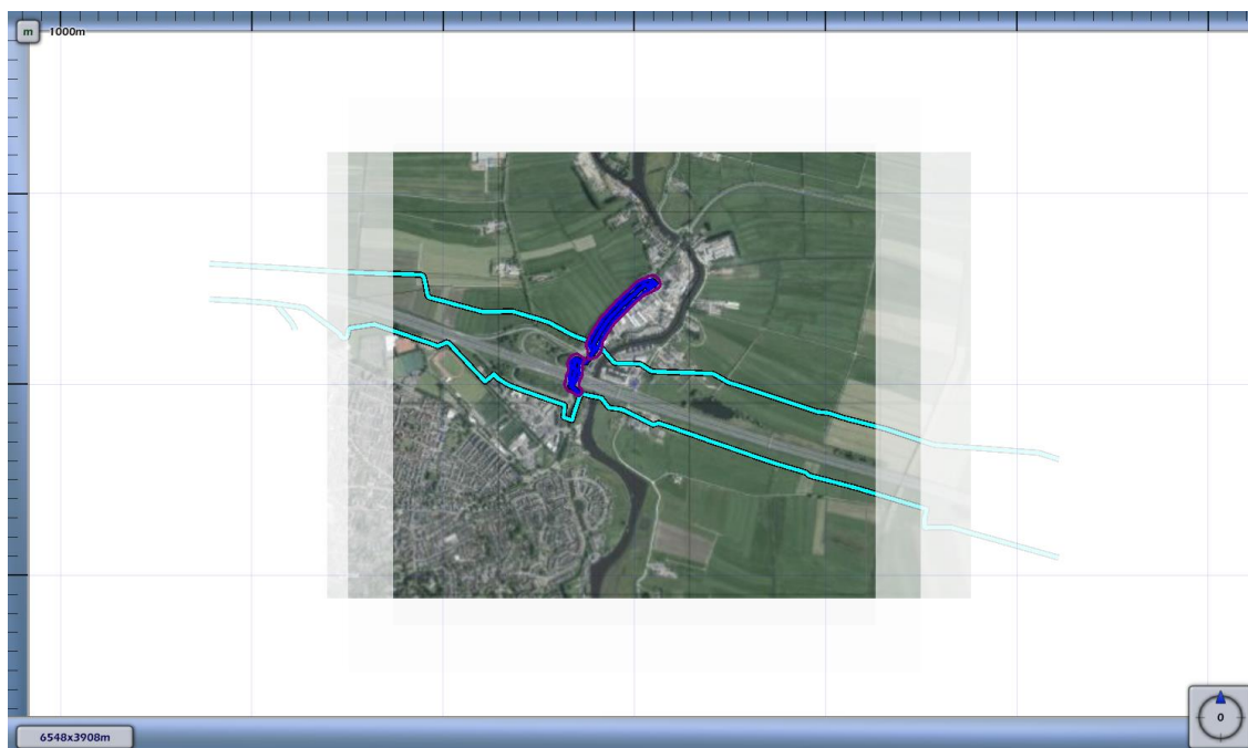
3.4 Figuur 3.4 Plaatsgebonden risico voor 8260_leiding-W-500-23-deel-1 van N.V. Nederlandse Gasunie
