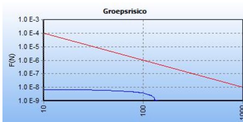
Afbeelding 12 fN-curve buisleiding W-500-01-deel-1, toekomstige situatie
