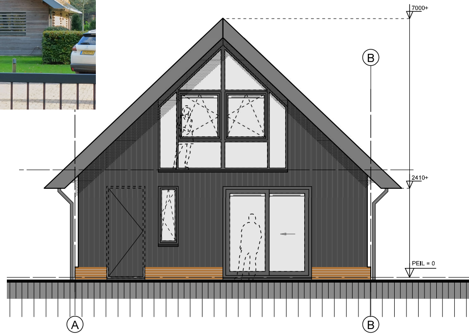
Achtergevel (oost)
