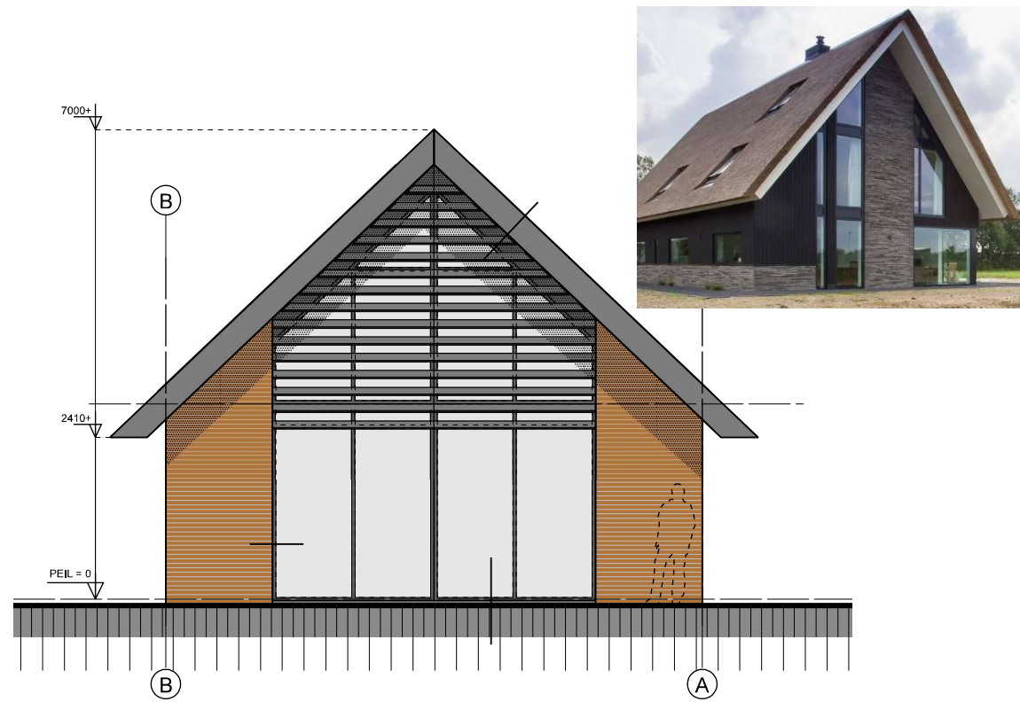
Voorgevel (west)
