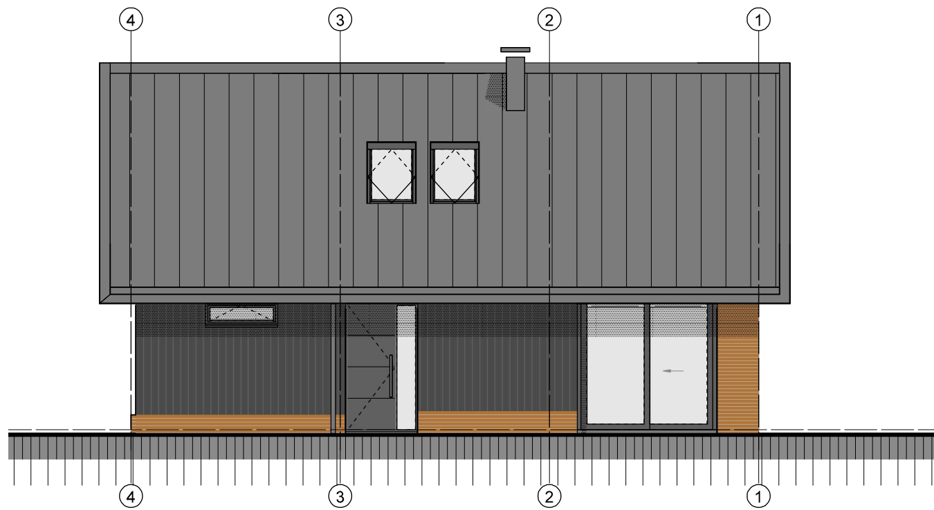
Linker zijgevel (noord)
