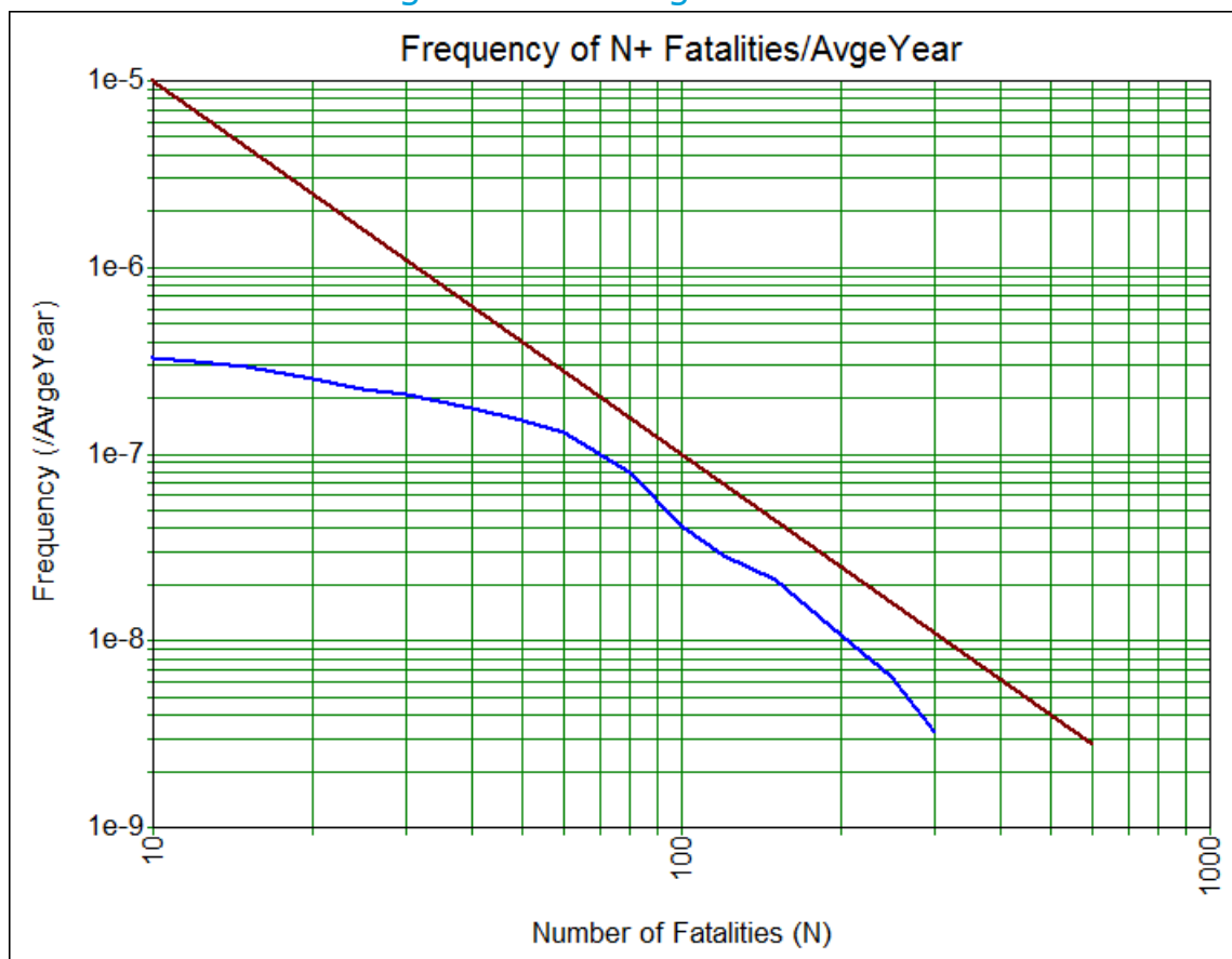
Figuur 7 Resultaat groepsrisicoberekening toekomstige situatie. De FN-curve is weergegevens door de blauwe lijn. De rode lijn geeft de oriëntatiewaarde aan.
