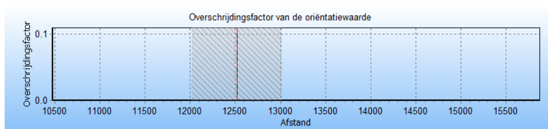
Figuur 19 Overschrijding van het groepsrisico als functie van de stationing van de W-500-01.
