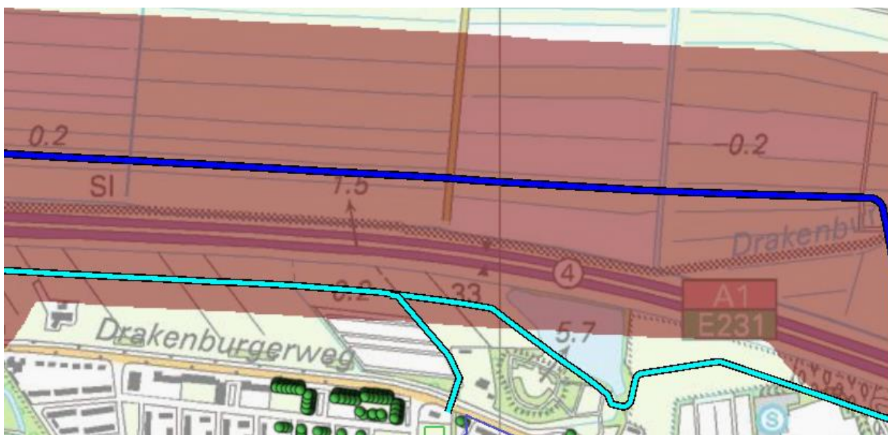
Figuur 9 Gastransportleiding A-510-01 met het invloedsgebied.
