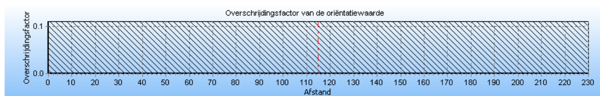
Figuur 13 Overschrijding van het groepsrisico als functie van de stationing van de W-500-23.
