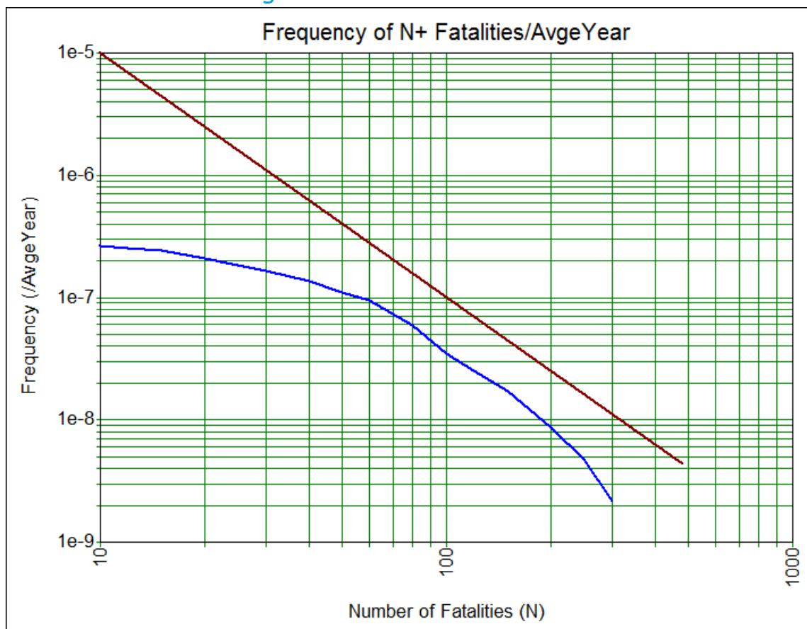
Figuur 6 Resultaat groepsrisicoberekening bestaande situatie. De FN-curve is weergegevens door de blauwe lijn. De rode lijn geeft de oriëntatiewaarde aan.
