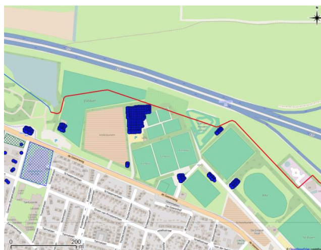
Figuur 20 FN curve van de kilometer met de hoogste overschrijdingsfactor 0.0 van de W-500-01. De ligging van de kilometer met de hoogste overschrijdingsfactor is hiernaast in het rood weergegeven op een topografische kaart.
