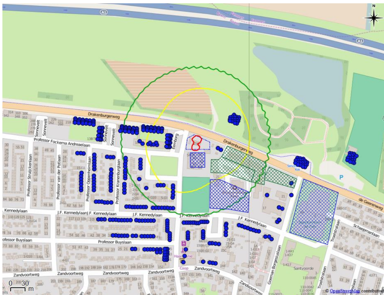
Figuur 5 Plaatsgebonden risicocontouren met faalfrequenties conform interim-regels RIVM van het gasontvangstation Baarn; contour voor het plaatsgebonden risico van 10^{-6} per jaar (rood), van 10^{-7} (geel) en van 10^{-8} (groen).
