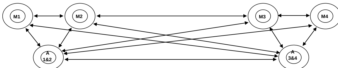
Figuur 4 Dwarsdoorsnede meetstraat GOS Baarn. De pijlen geven aan tussen welke leidingen escalatie van lek naar breuk kan plaatsvinden. De bovenste leidingen (M1, M2, M3 en M4) zijn de meetstraten en de onderste leidingen (A1&2 en A3&4) zijn de aanvoerleidingen.
