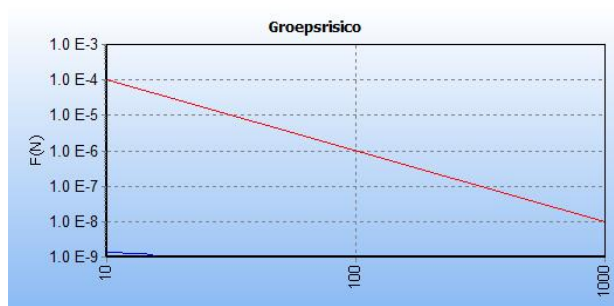
Figuur 16 FN curve van de kilometer met de hoogste overschrijdingsfactor 0.0 van de W-500-23. De ligging van de kilometer met de hoogste overschrijdingsfactor is hiernaast in het rood weergegeven op een topografische kaart.
