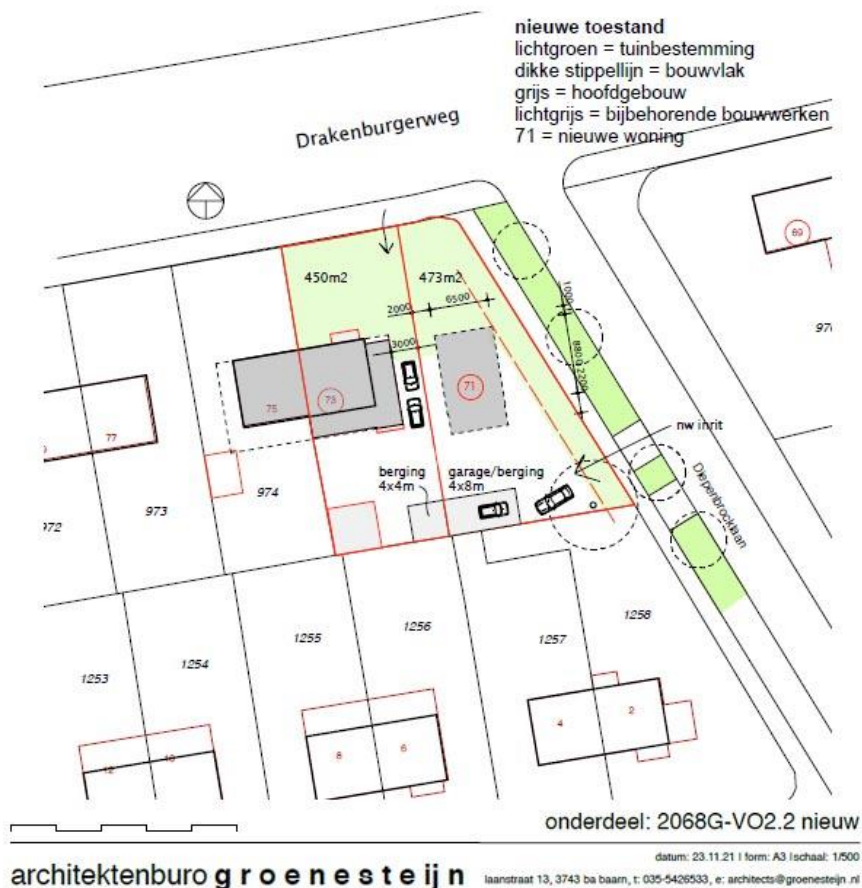
Figuur 1 voorlopig ontwerp voor perceel Drakenburgerweg 73 in Baarn
